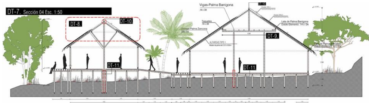
Figura 32: Corte funcional
