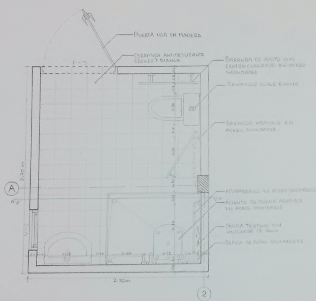
BAÑO DISCAPACITADO TIPO ESC. 1:20
