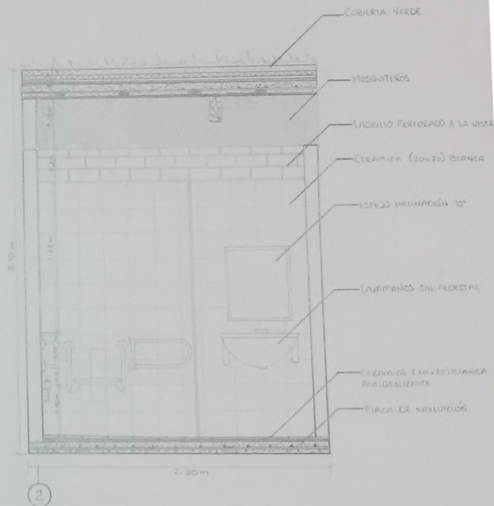
CORTE A-A' ESC. 1:20
