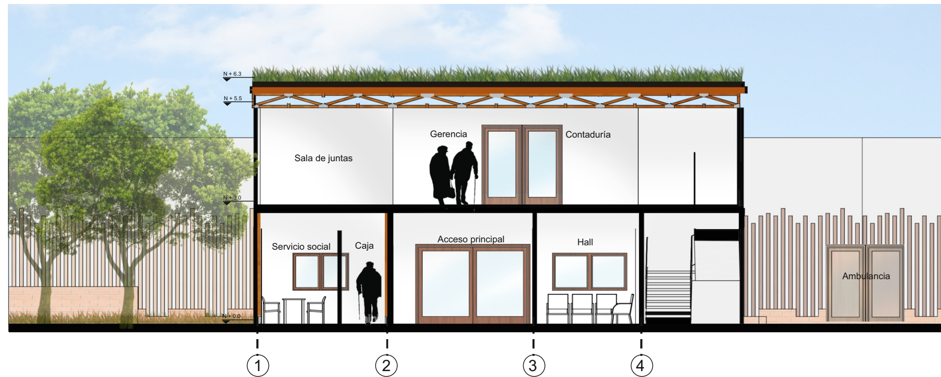
CORTE ADMINISTRACIÓN / ESC. 1:100
