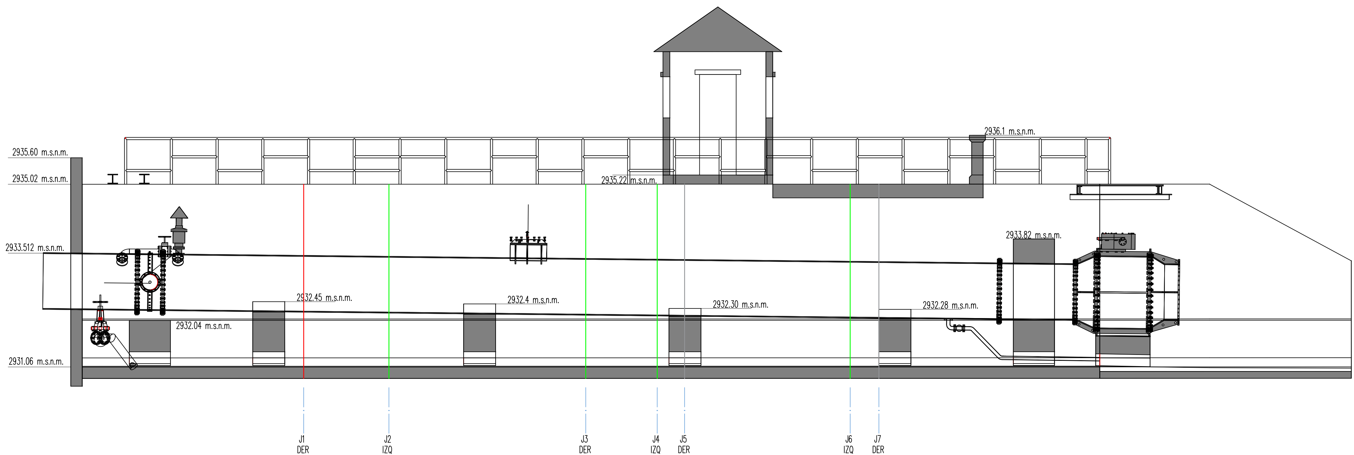
PERFIL LONGITUDINAL CANAL DE DESCARGA Escala 1:50
