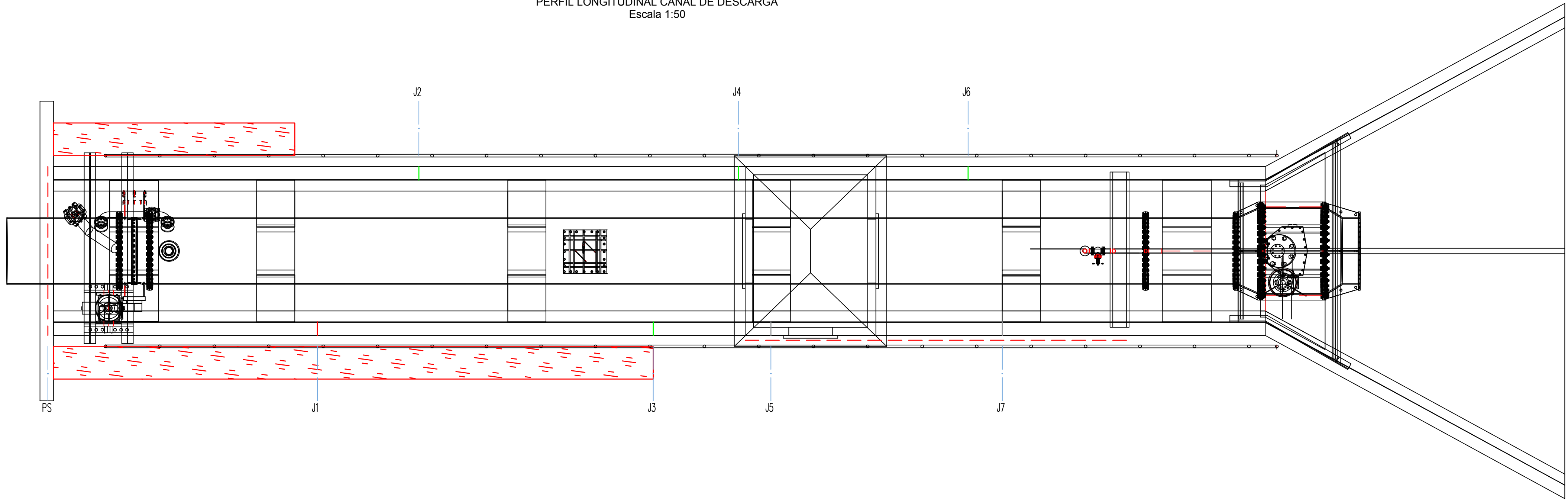
PLANTA GENERAL CANAL DE DESCARGA Escala 1:50
