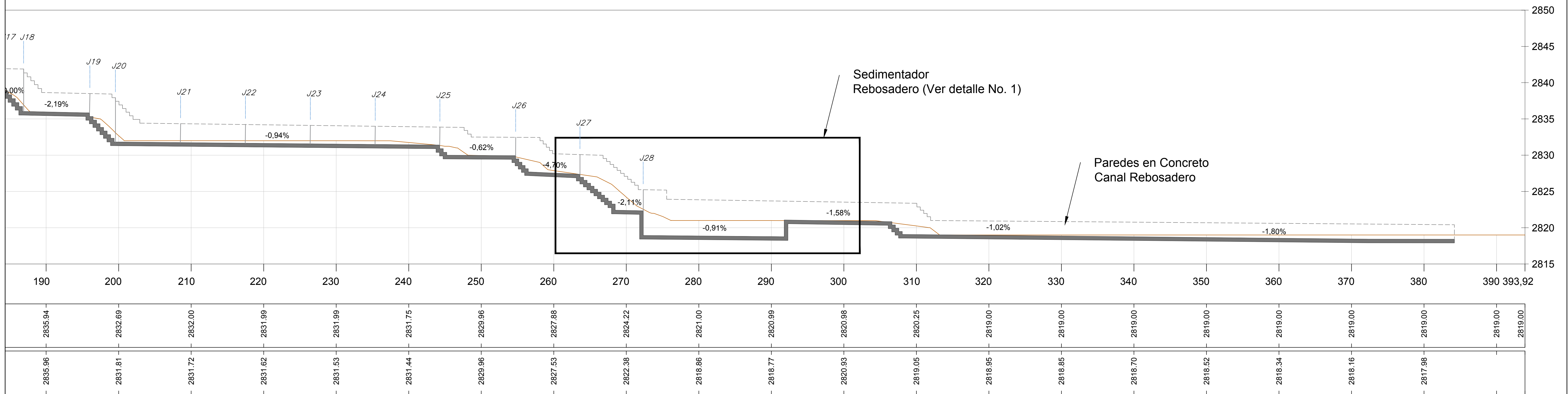
PERFIL LONGITUDINAL REBOSADERO EL HATO Escala 1:250
