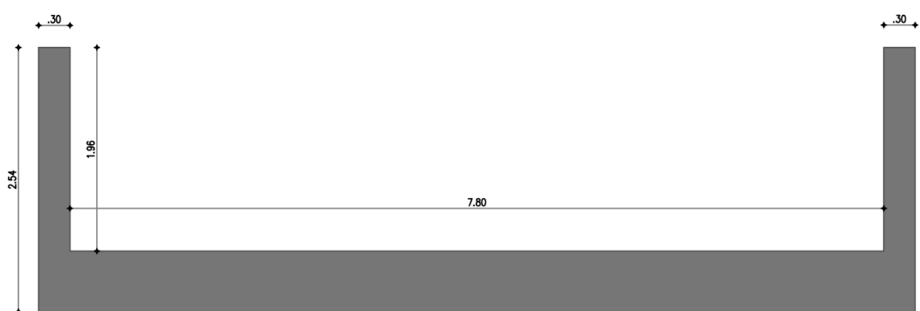
CORTE C-C' Escala 1:50
