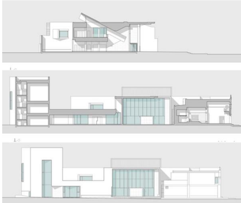
Figura 36. Fachadas. Tipología 2. Biblioteca municipal de Ílhavo / ARX Portugal
