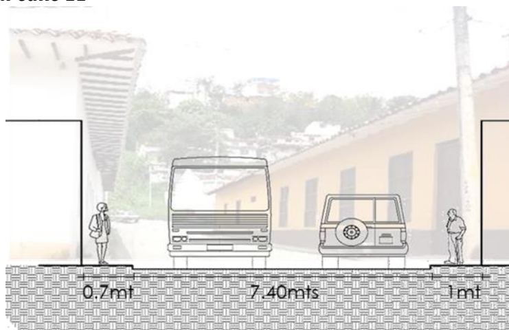
Figura 22. Perfil actual calle 11
