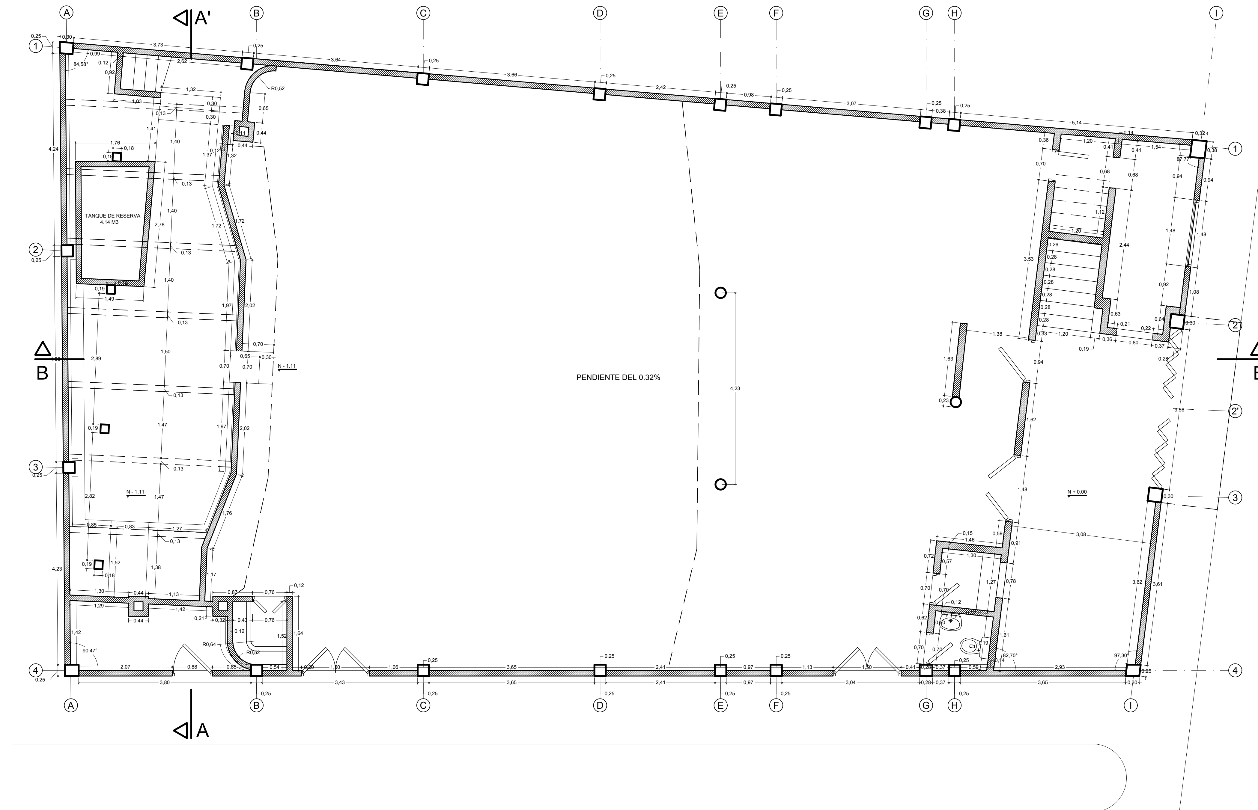
PLANTA SEMISOTANO Y PRIMER PISO
