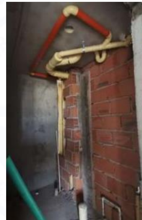
Proyecto Arboleda Campestre 4 Supervisión pruebas hidrosanitarias torre 2 Fuente: Propia
