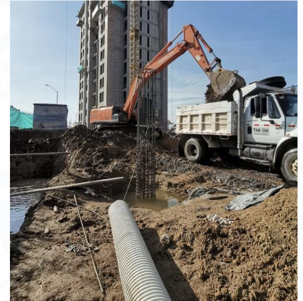
Proyecto Arboleda Campestre 4 Excavación mecánica plataforma vehicular Fuente: Propia
