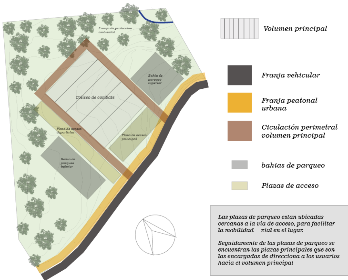
Figura 22. Imagen: Esquema funcional implantación y zonificación urbana
