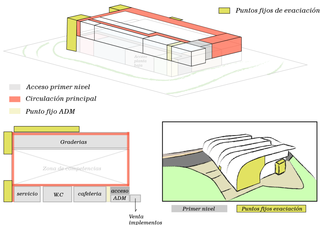
Figura 27. Esquema circulación y salidas de emergencia planta primer nivel
