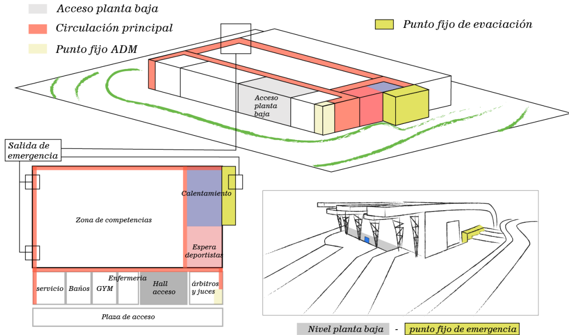
Figura 26. Esquema circulación y salidas de emergencia planta baja
