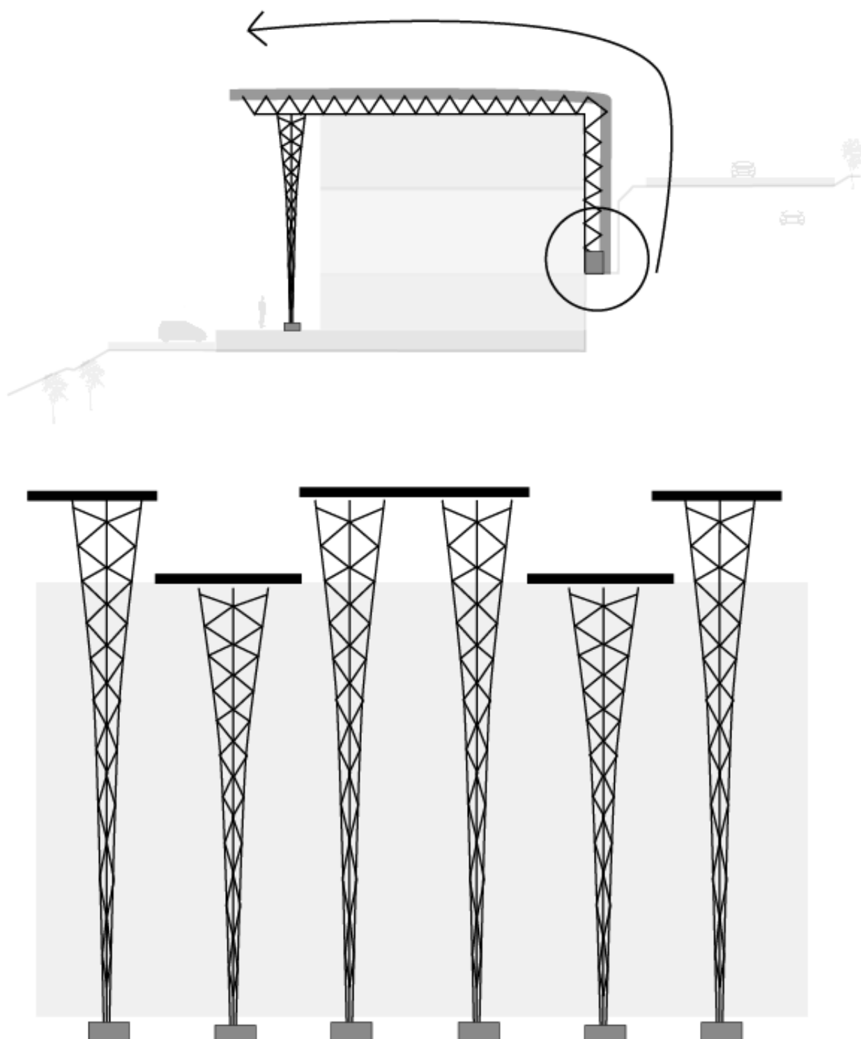
Figura 31. Representación estructura de cubierta
