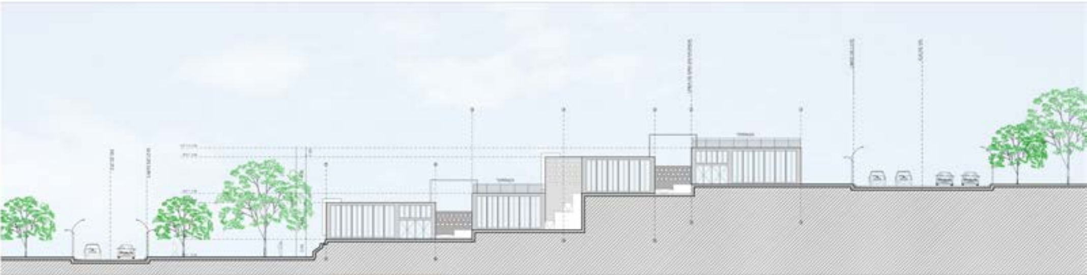
Figura 44. Mejía, Néstor. Fachada Lateral, 2018. Maceo - Antioquia.
