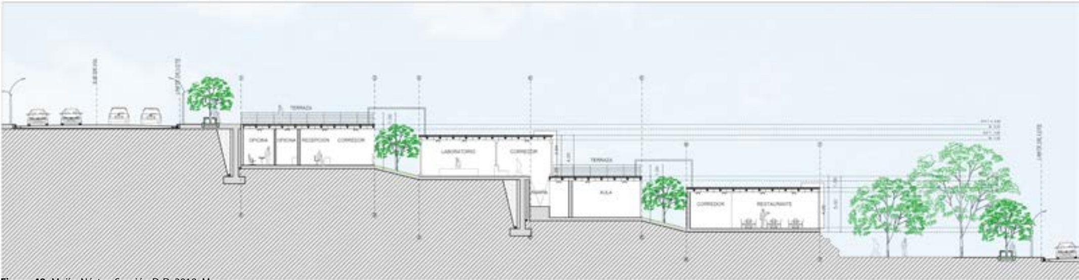
Figura 48. Mejía, Néstor. Sección D-D, 2018. Maceo - Antioquia.
