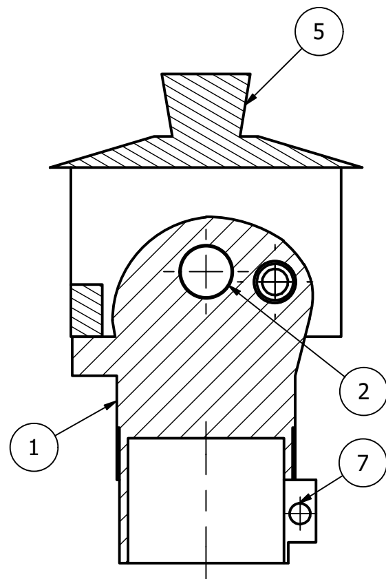
SECCIÓN D-D ESCALA 1 : 1
