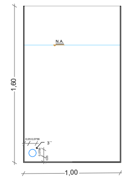
CORTE E-E
