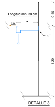
DETALLE 3
