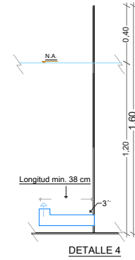
DETALLE 4
