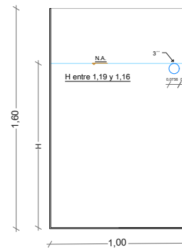
CORTE D-D
