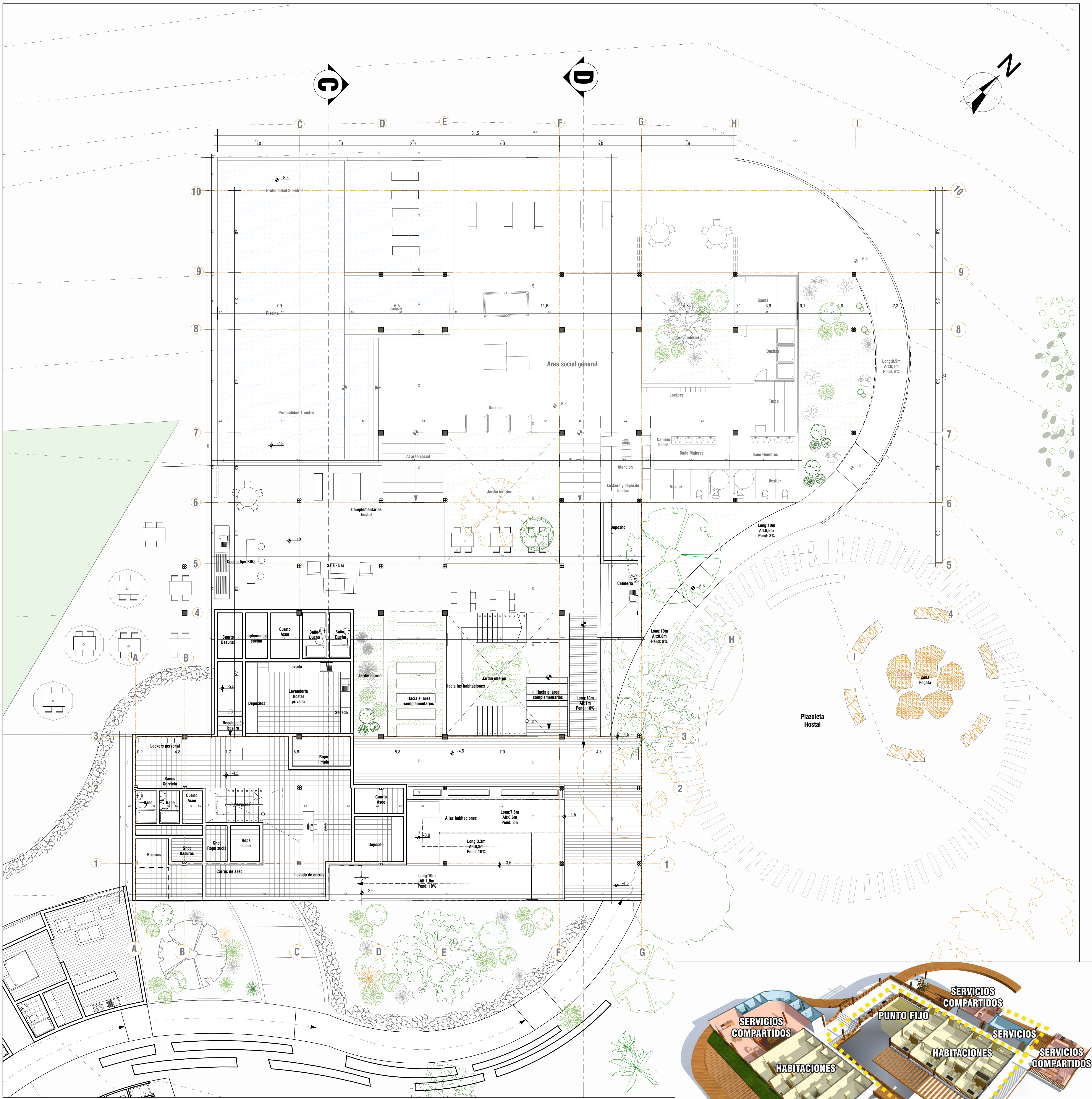
Planta Baja Bloque B Esc_1:100
