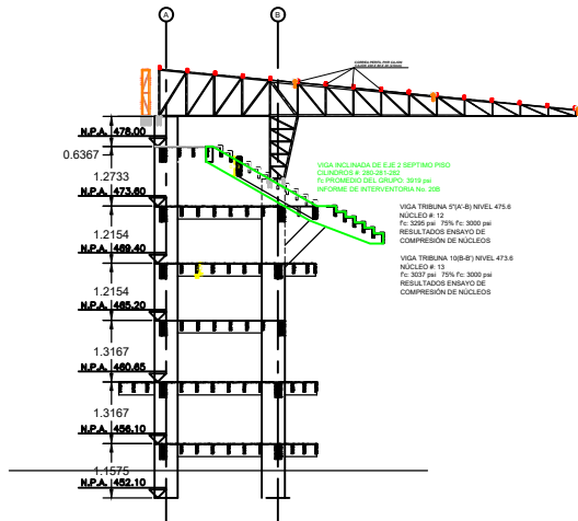
CORTE ESTRUCTURAL EJE 2 CORTE 2-2
