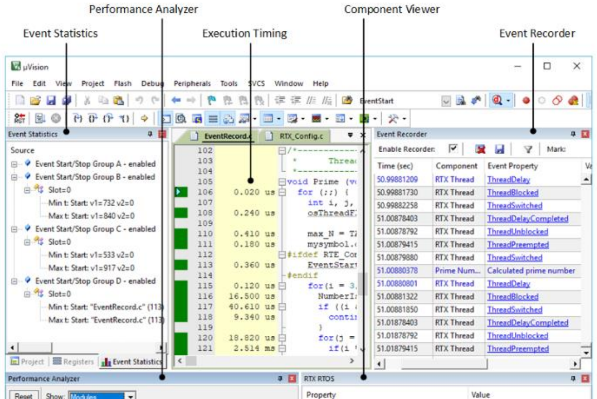
FIGURA 6.13 KEIL UVISION DEBUGGER
