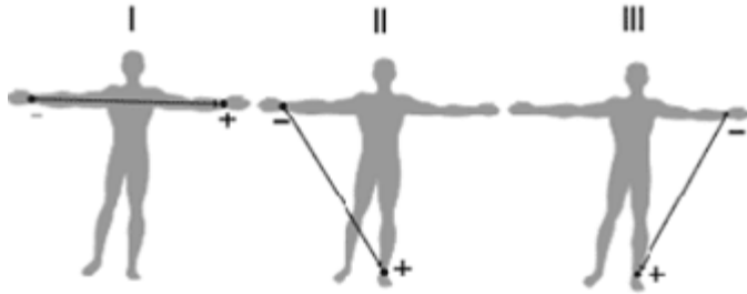
FIGURA 5.4 DERIVACIONES BIPOLARES
