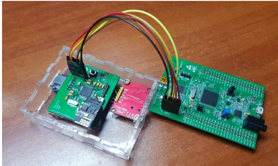
FIGURA 6.8 STM32F407VG COMO PROGRAMADOR CONECTADO AL MICROCONTROLADOR DISEÑADO
