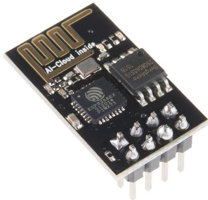
FIGURA 6.6 MODULO ESP01
