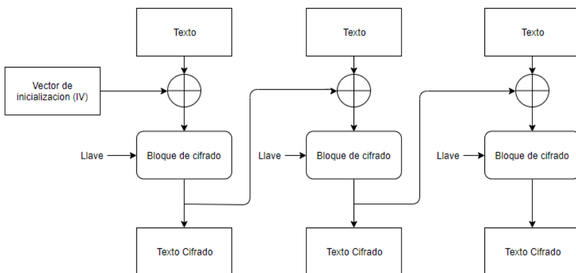
FIGURA 5.9 CIFRADO POR BLOQUES CBC
