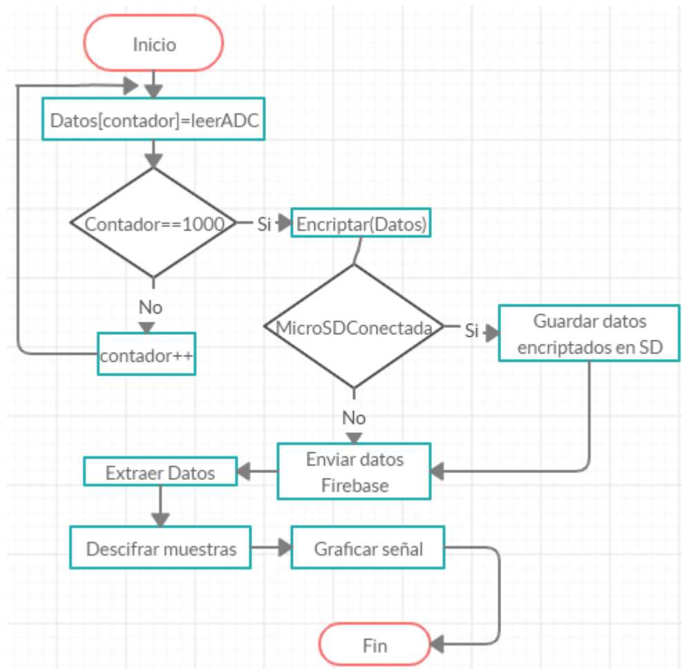
FIGURA 7.11 DIAGRAMA DE FLUJO DEL SISTEMA DE PROGRAMACIÓN
