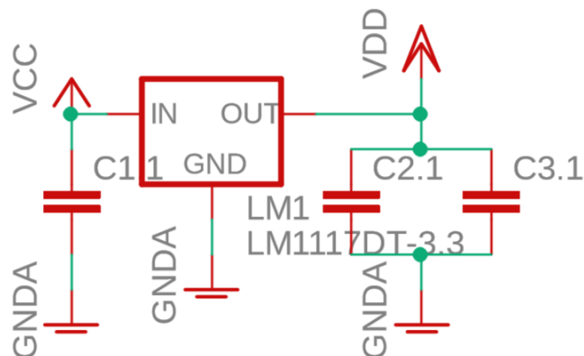
FIGURA 6.9 ALIMENTACIÓN DEL SISTEMA
