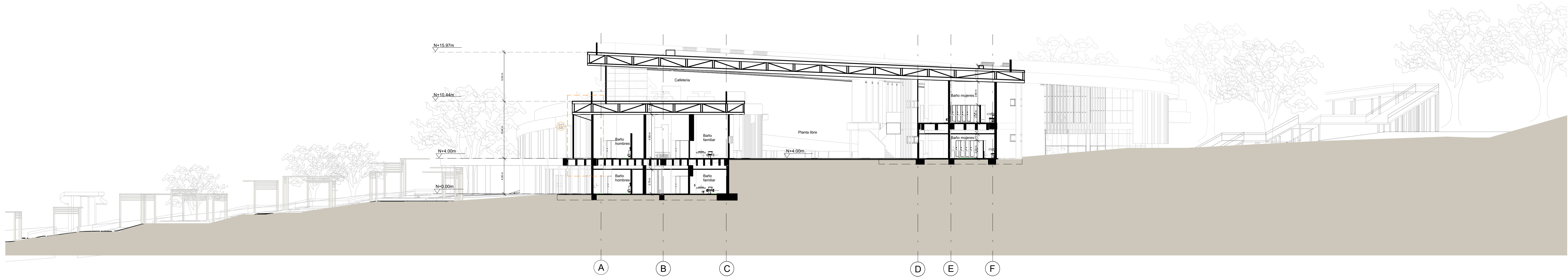
CORTE TRANSVERSAL C-4 Esc 1.200
