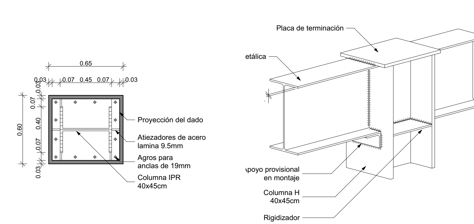
Union de columnas con cimentación
