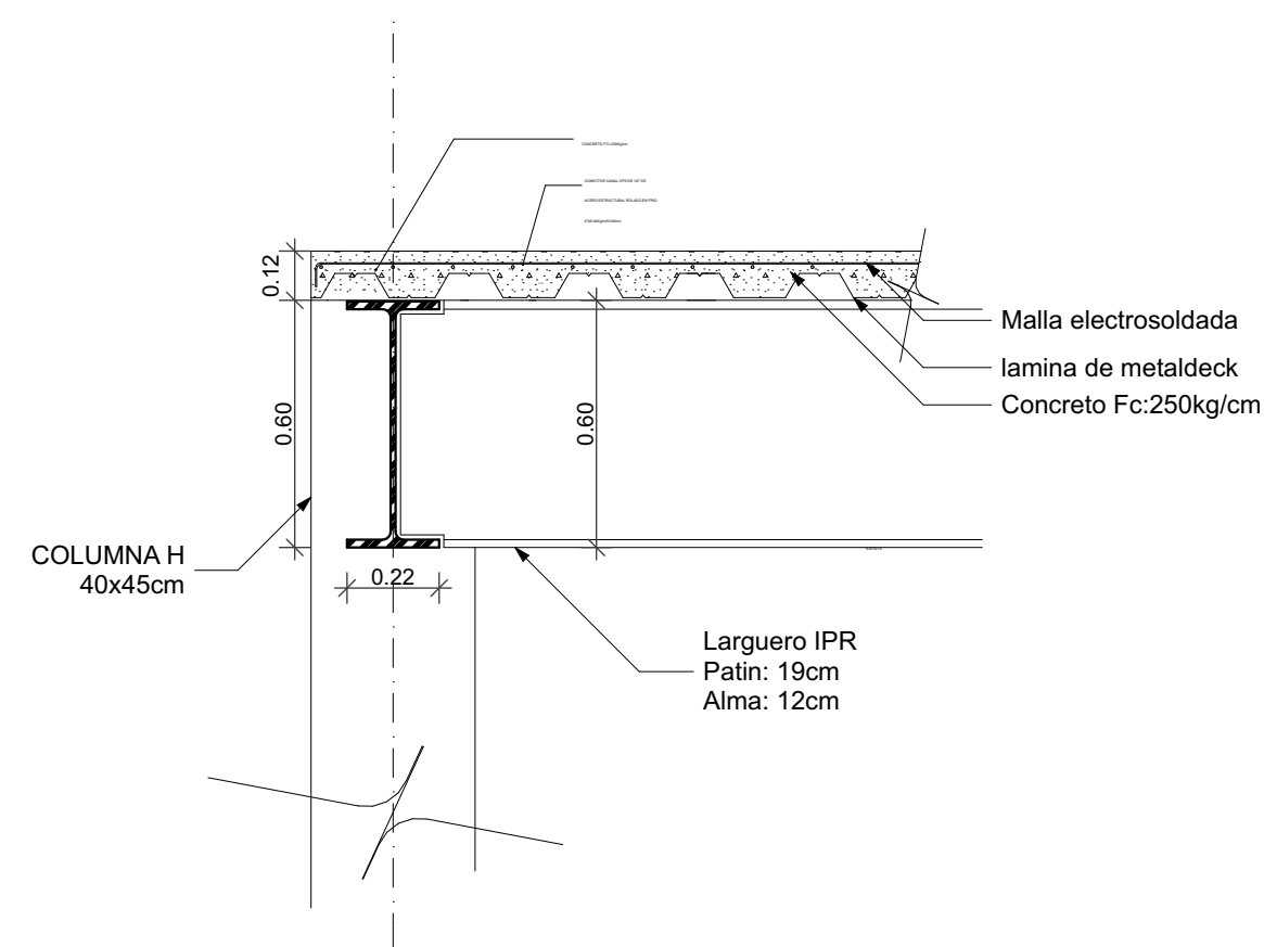
Sistema de entrepiso: Metaldeck
