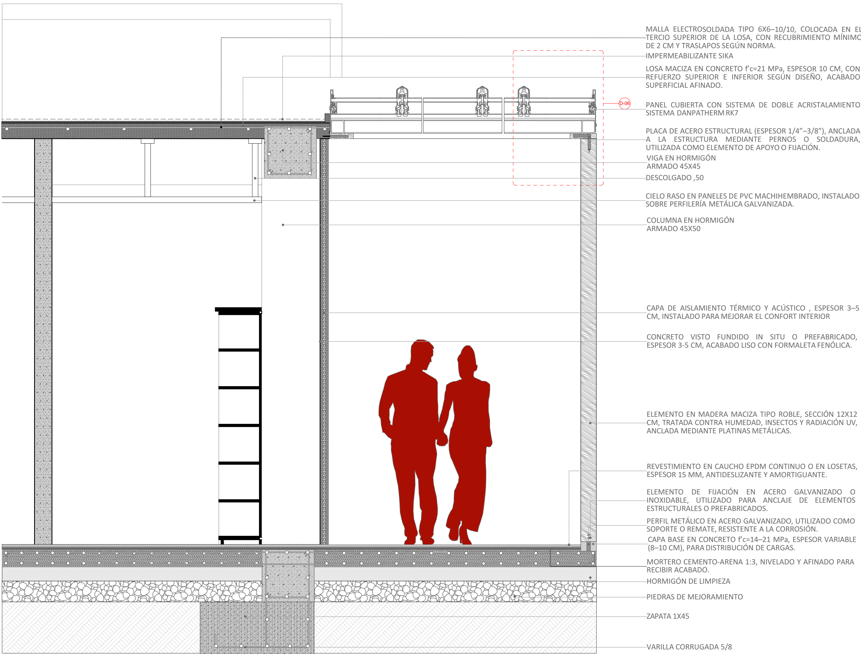
CORTE FACHADA D03
