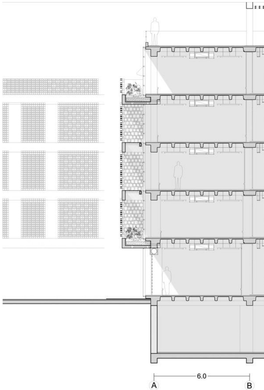
Figura 34. Corte C-C'.
