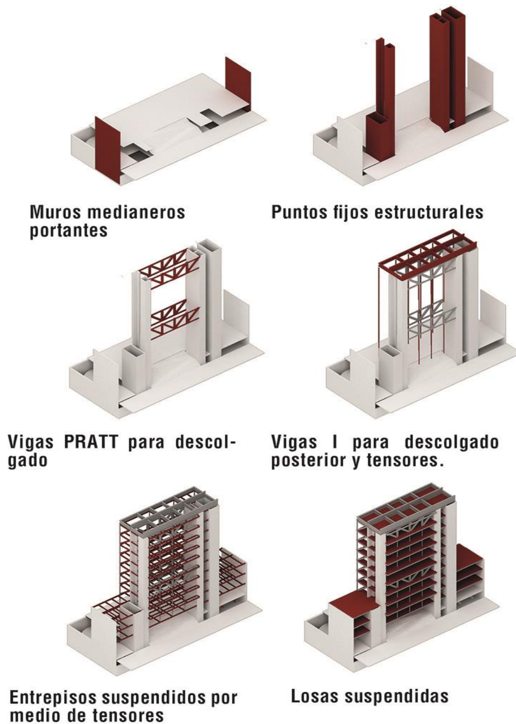
Figura 25. Sistema Estructural.
