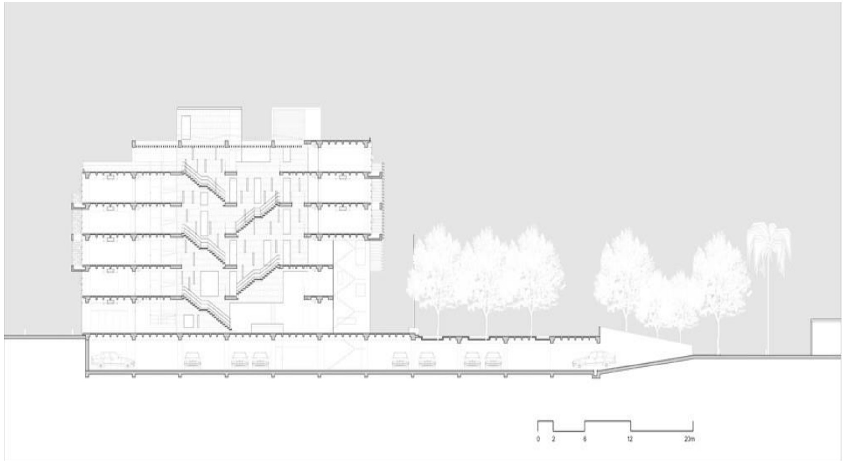
Figura 32. Corte A-A'.
