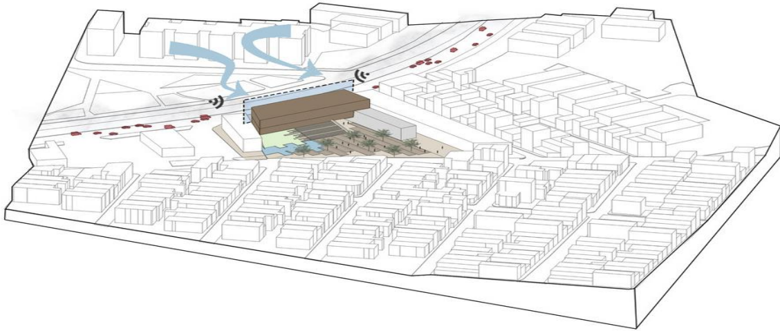
Figura 53. Ventilación.
