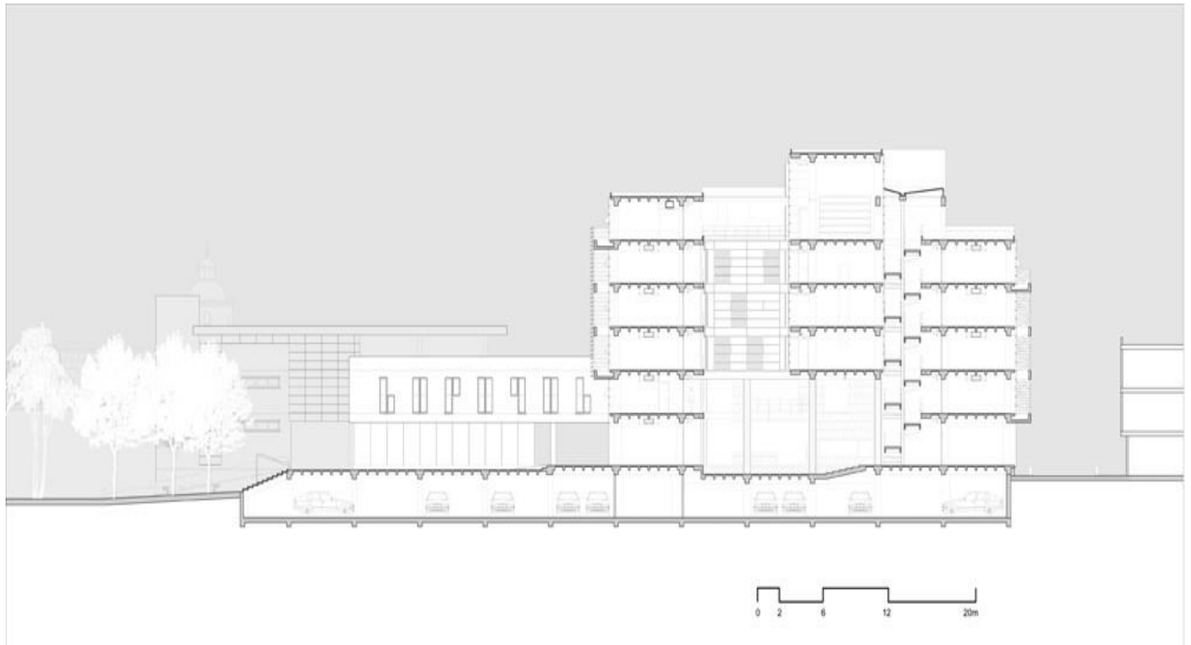
Figura 33. Corte B-B'.
