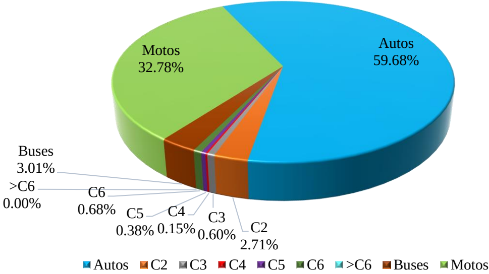
Porcentaje de vehiculos en la hora de máxima demanda ramal G
