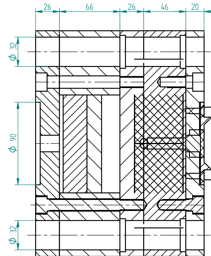
SECTION A-A
