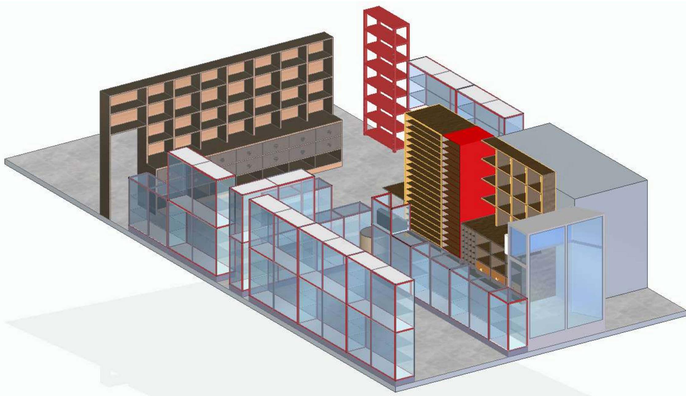
Grafico 1 Vista 3D distribución Almacén Verona
