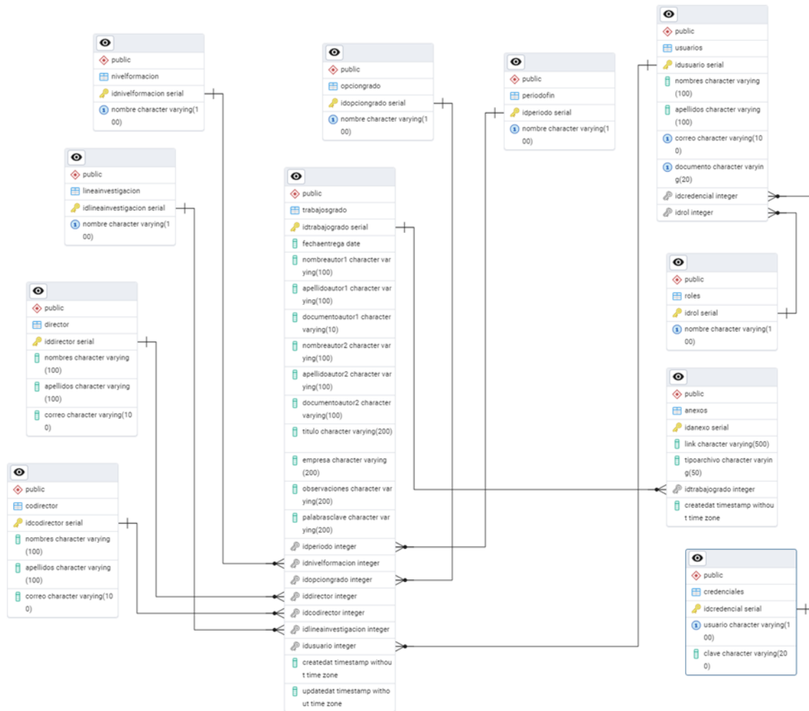
Figura 8. Esquema relacional de la base de datos
