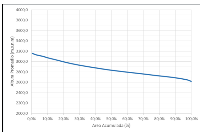
Figura 1-3 Curva hipsométrica, Cuenca Varguitas Fuente. Consorcio Aguas de los Andes
