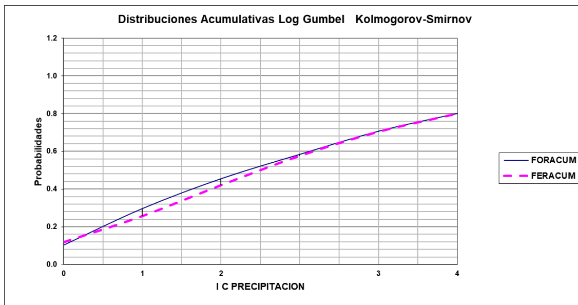
Figura 3-20 Análisis estadístico, ajustes de distribuciones extremos.
