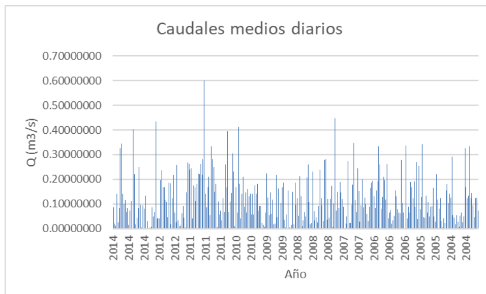
Figura 3-13 Caudales medios estimados, para la cuenca Varguitas Fuente. Consorcio Aguas de los Andes, 2018
