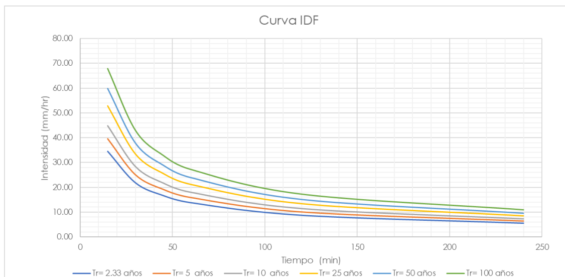
Figura 3-2 Curvas IDF, estación Tunguavita Fuente: Consorcio Aguas de los Andes, 2018
