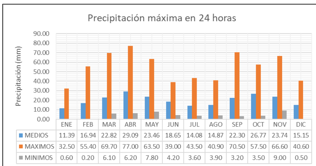
Figura 2-2 Valores máximos, medios y mínimos mensuales de precipitación Fuente. Consorcio Aguas de los Andes, 2018
