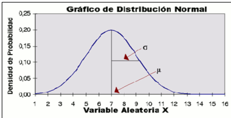
Figura 3-16 Distribución Normal
