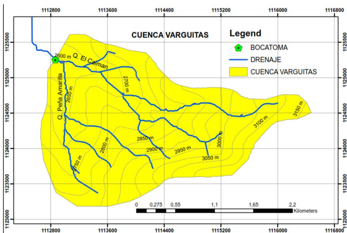
Figura 1-2 Delimitación de la cuenca, Varguitas Fuente. Consorcio Aguas de los Andes, 2018
