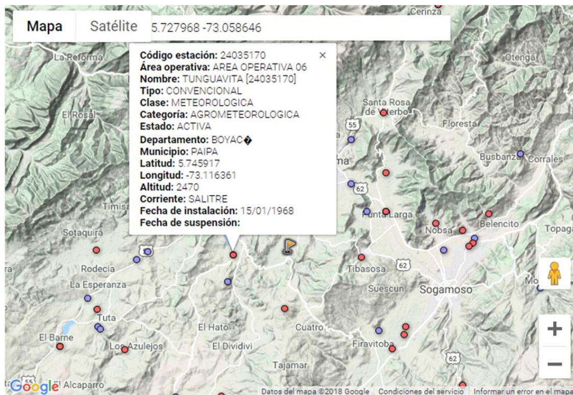
Figura 2-1 Distribución espacial de las estaciones Fuente. Consorcio Aguas de los Andes, IDEAM, 2018
