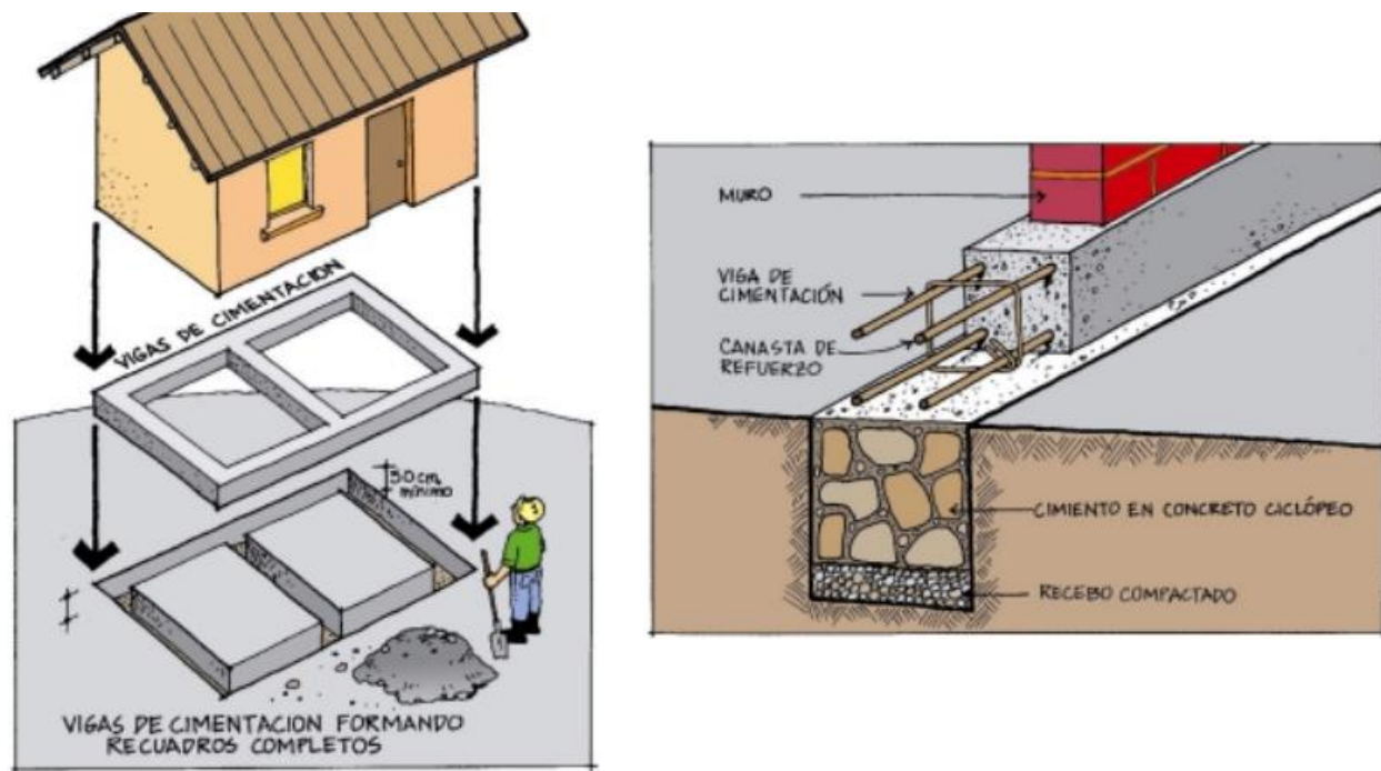
Figura 10. Principales aspectos a tener en cuenta a la hora de utilizar como Sistema constructivo la mampostería confinada. Adaptado de Asociación Colombiana de Ingeniería Sísmica, 2001. Disponible en la página web La Red, sitio web: http://www.desenredando.org .
