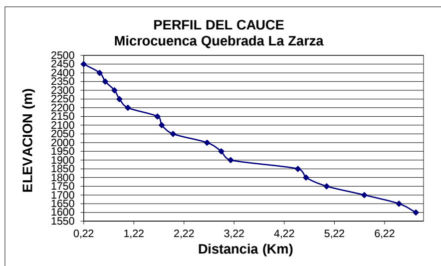
Figura 4. Perfil Microcuenca Quebrada La Zarza, adaptado del EOT El Guacamayo, 2014
