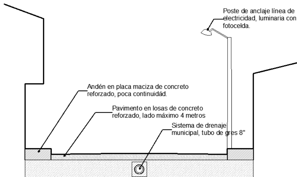
Figura 12. Alzado general de una calle o en el municipio de El Guacamayo.
