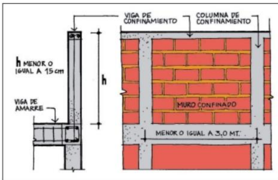
Figura 9. Esquema general de funcionamiento del Sistema de construcción en mampostería confinada, Adaptado de Asociación Colombiana de Ingeniería Sísmica, 2001. Disponible en la página web La Red, sitio web: http://www.desenredando.org .
