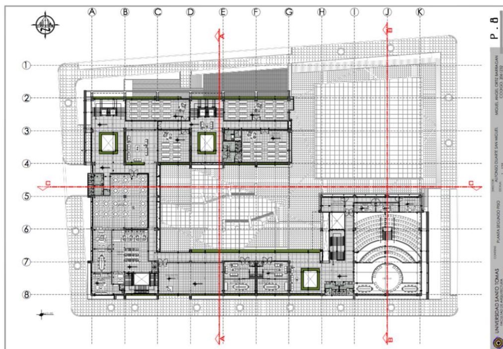
Apéndice I Planta Segundo Piso
