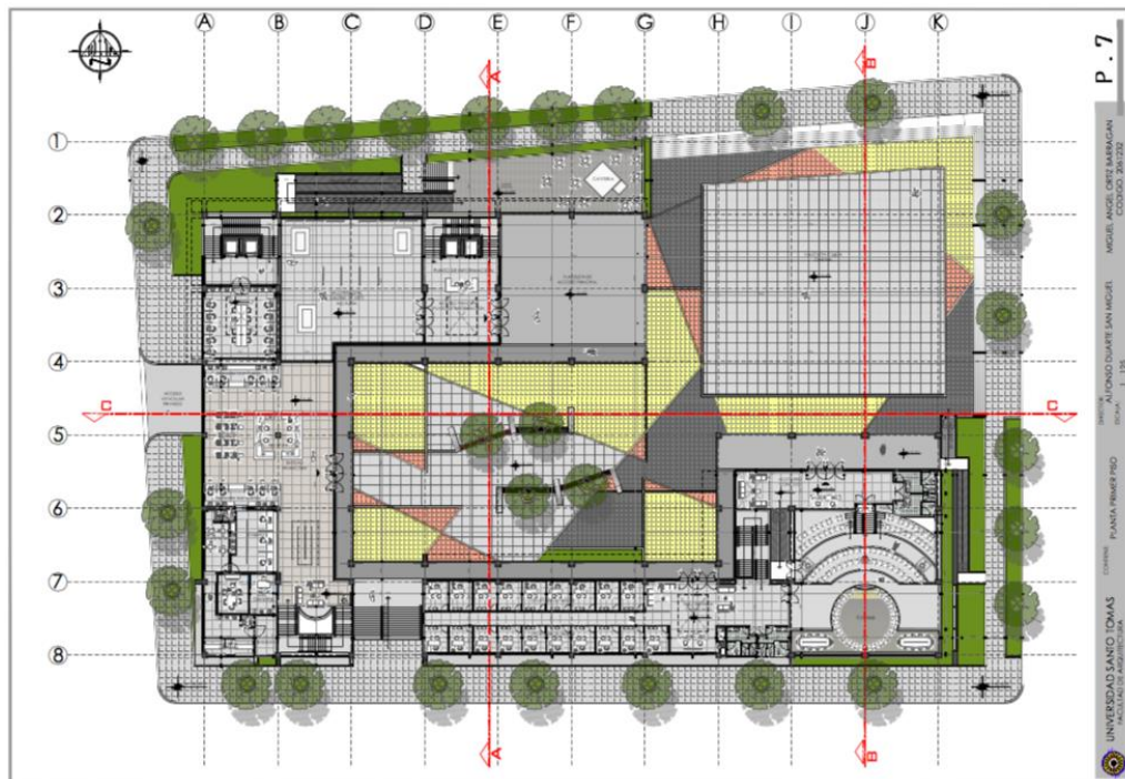
Apéndice H Planta Primer Piso
