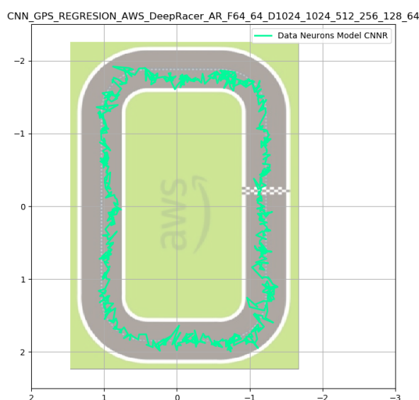
(A) Trayectoria obtenia por la CNN del modelo #8.
