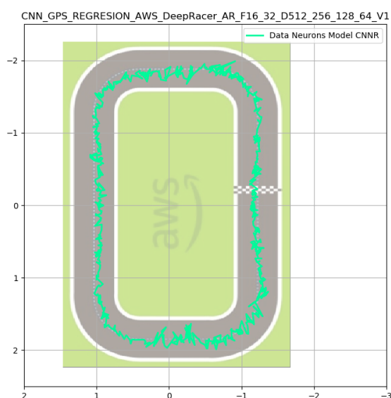
(A) Trayectoria obtenia por la CNN del modelo #4.
