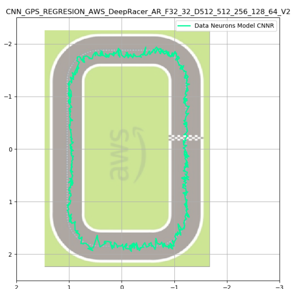
(A) Trayectoria obtenia por la CNN del modelo #5.
