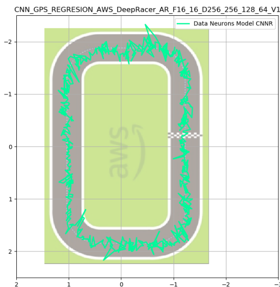
(A) Trayectoria obtenia por la CNN del modelo #3.
