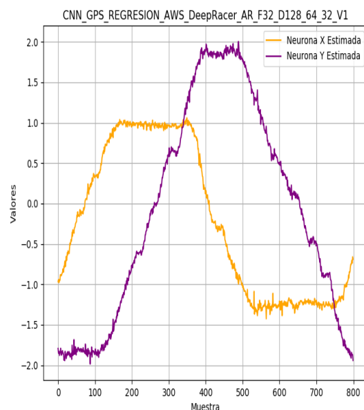
(B) Coordenadas X e Y estimadas.
