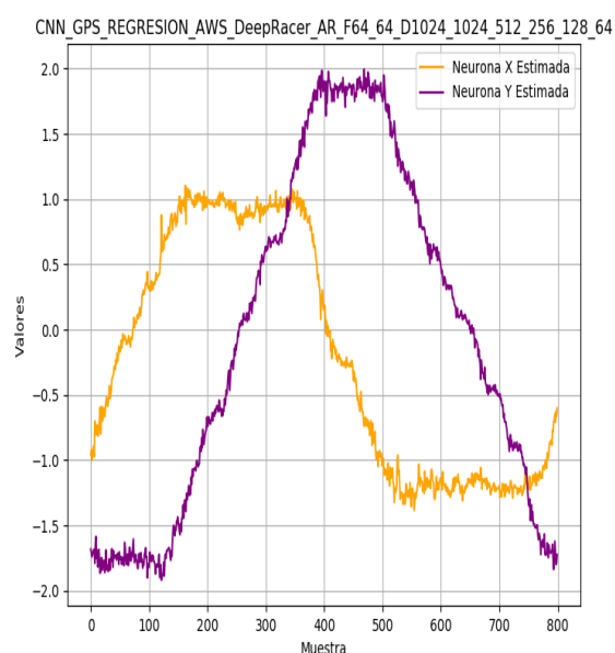
(B) Coordenadas X e Y estimadas.
