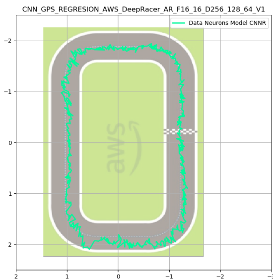
(A) Trayectoria obtenia por la CNN del modelo #2.
