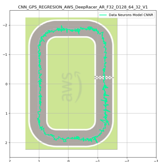
(A) Trayectoria obtenia por la CNN del modelo #7.
