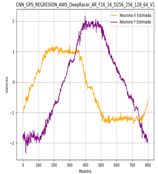
(B) Coordenadas X e Y estimadas.
