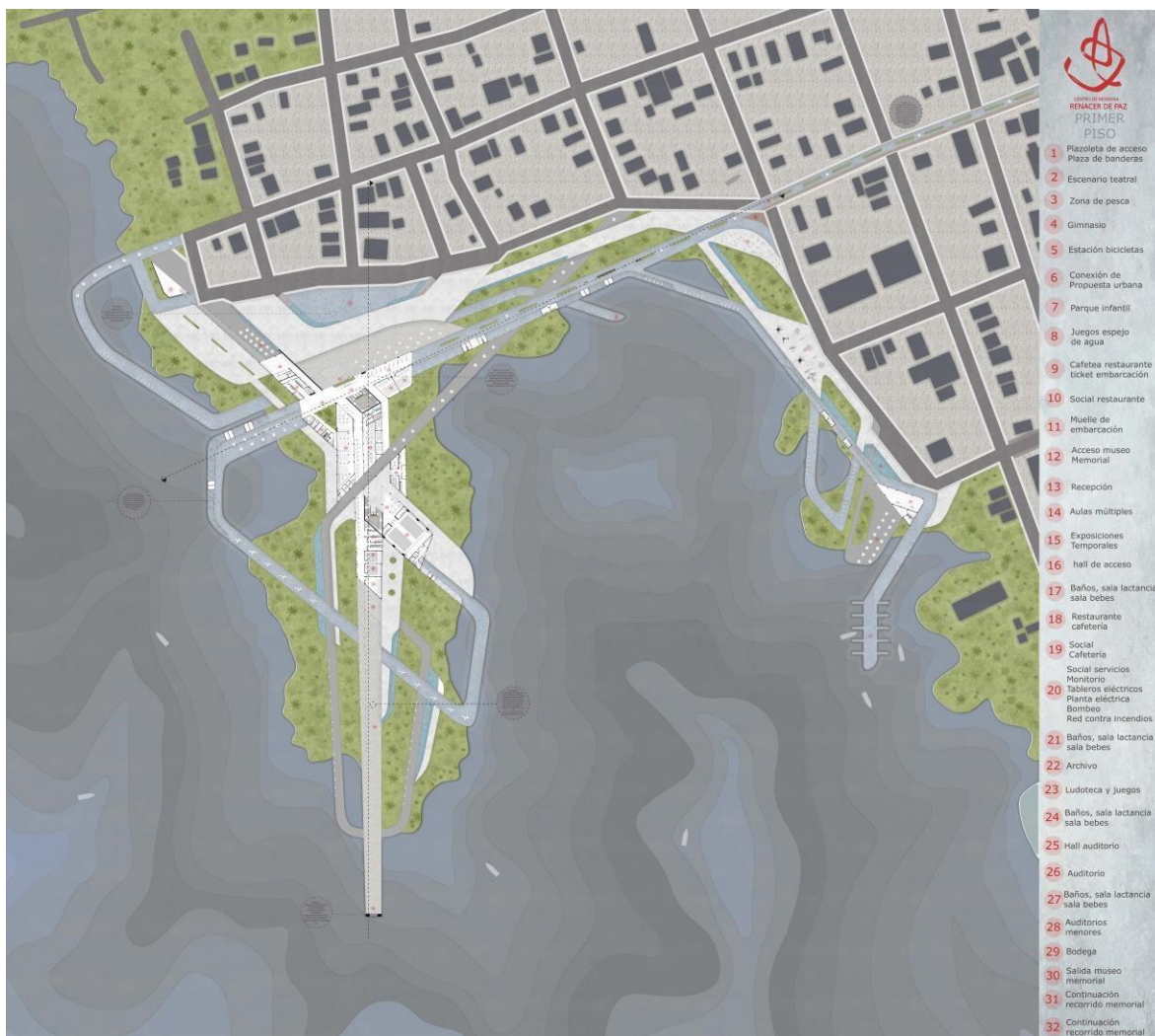
Ilustración 30. Planta primer piso
