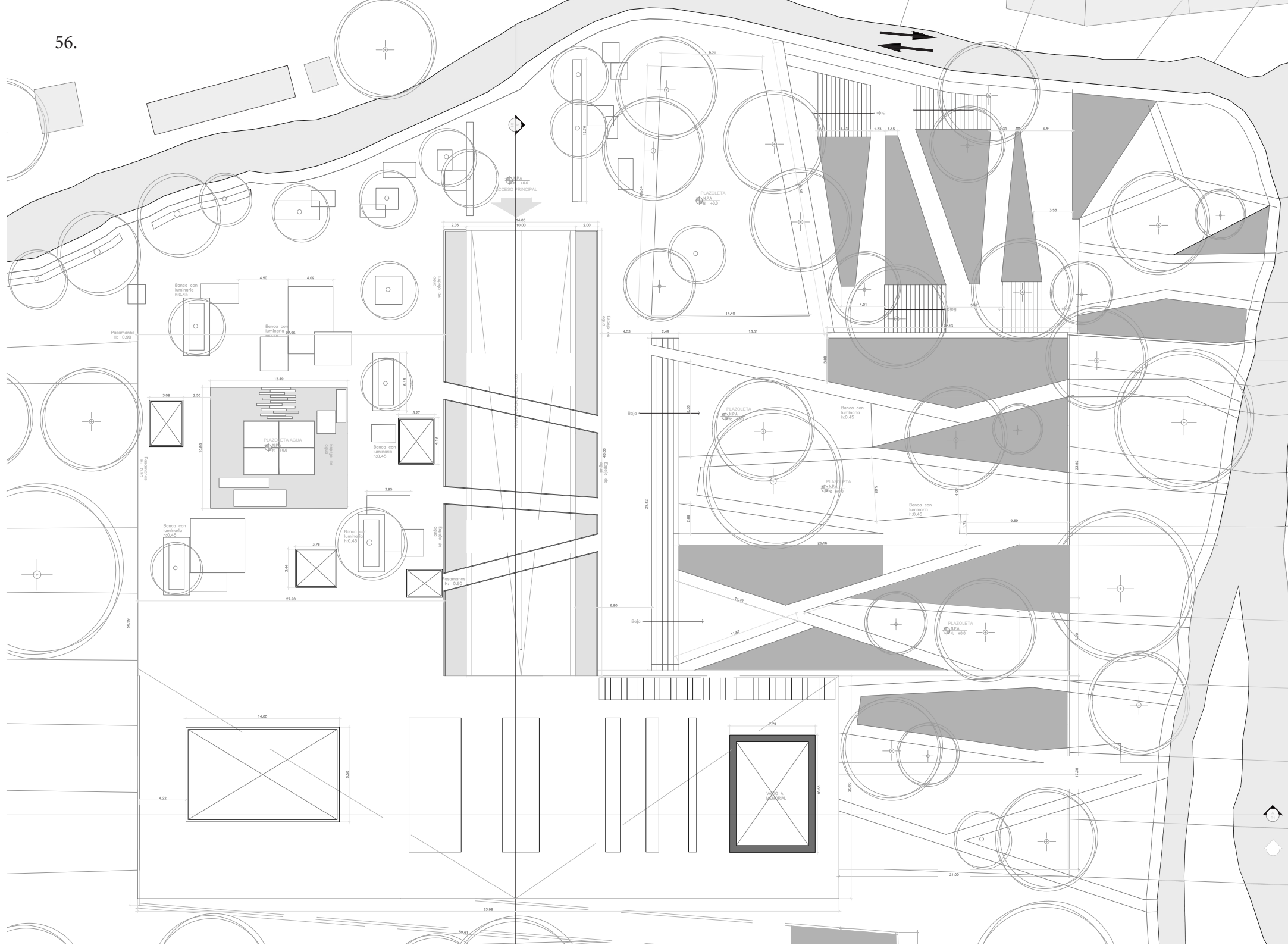
Figura 22. PLANTA PRIMER NIVEL.
