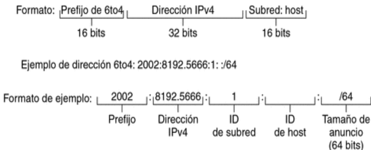
Imagen 4 Formato de direcciones IPv6
