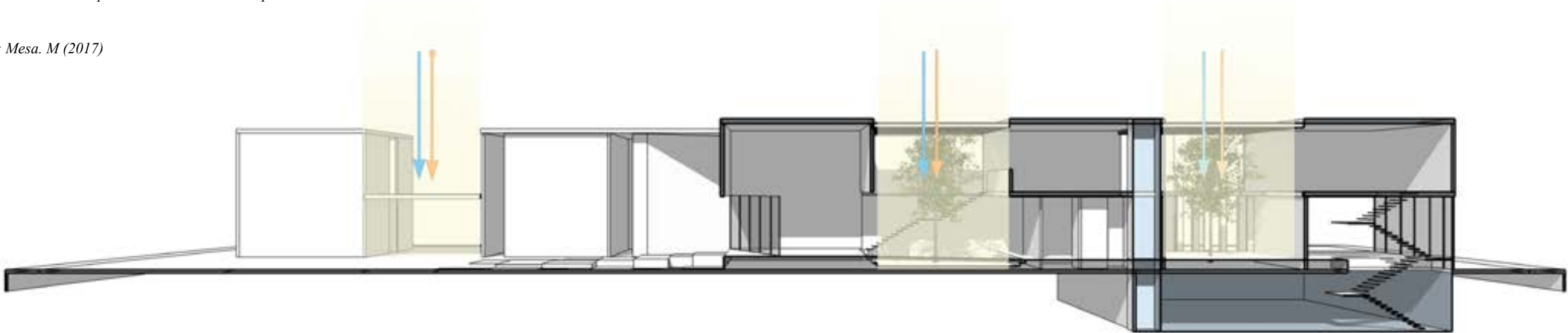
Figura 39: Primeros acercamientos en sección a la materialización del mecanismo espacial.
