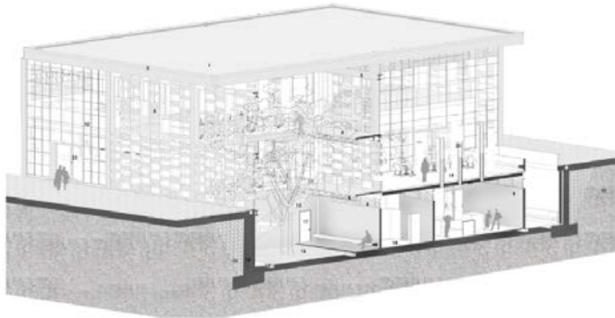
Figura 52: Perspectiva de detalle constructivo
