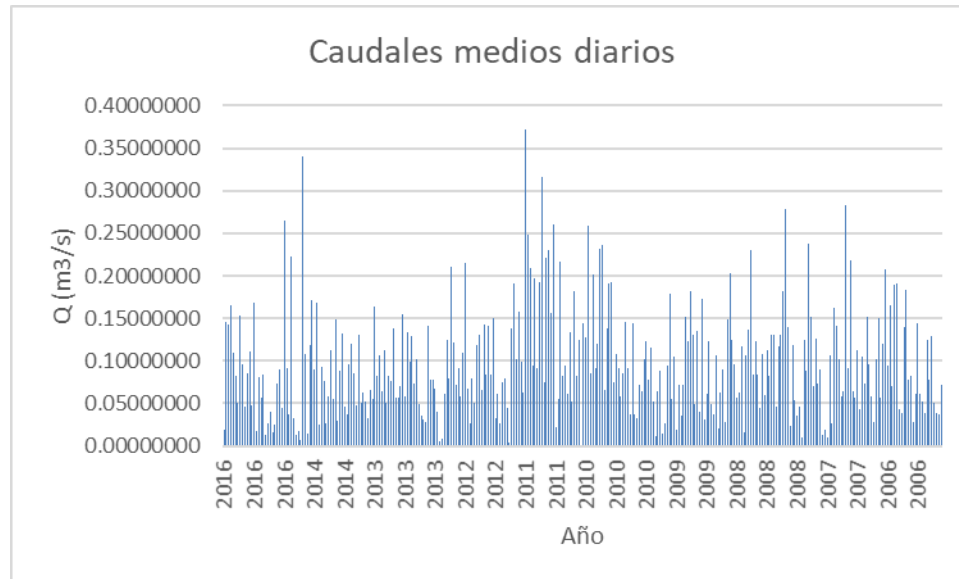
Figura 3-13 Caudales medios estimados, para la cuenca Nacupay Fuente. Consorcio Aguas de los Andes, 2018
