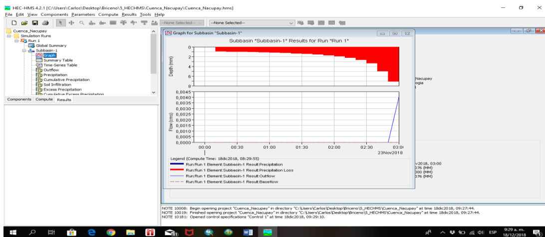
Figura 3-10 Hidrograma y curva de caudal Fuente. Consorcio Aguas de los Andes, 2018
