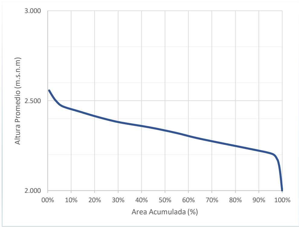
Figura 1-3 Curva Hipsométrica Fuente. Consorcio Aguas de los Andes, 2018
