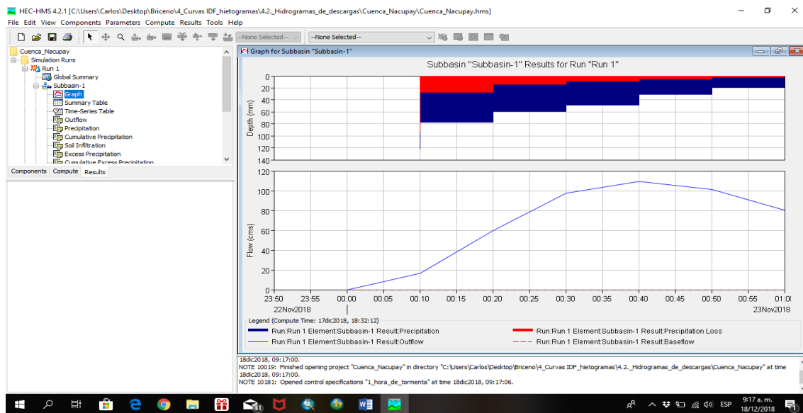
Figura 3-3 Hietograma e hidrograma de descarga 1 hora de tormenta Fuente. Consorcio Aguas de los Andes, 2018
