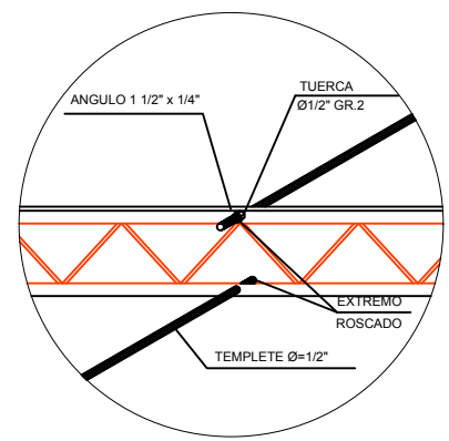
DETALLE
