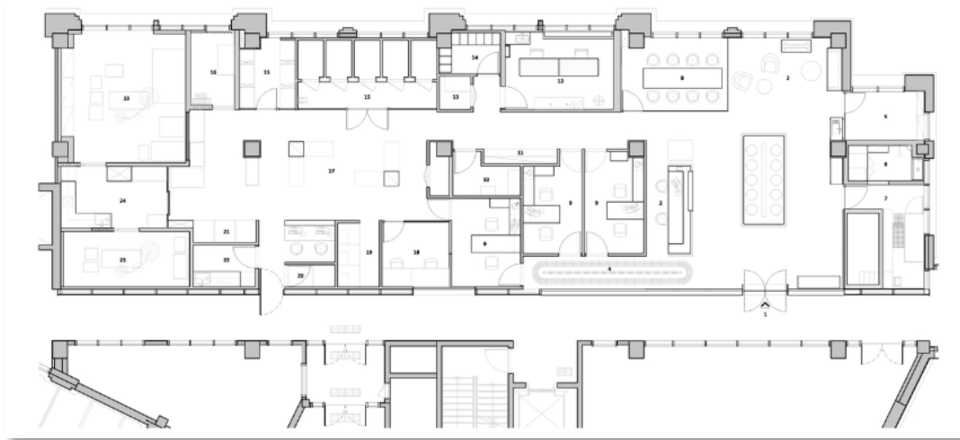
Figura 9. Planta general (Oasis veterinary (centro clínico – veterinario))
