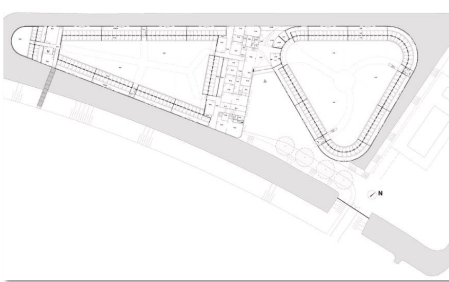
Figura 1. Planta general (centro de protección para animales)
