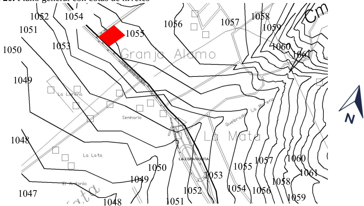
Figura 20. Plano general con cotas de niveles
