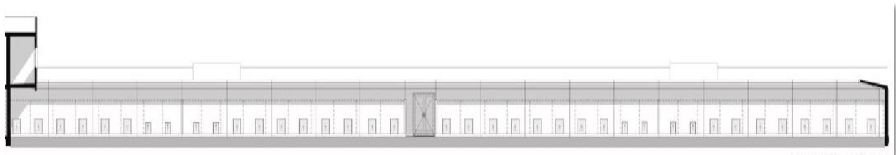
Figura 2. Corte longitudinal (centro de protección para animales)
