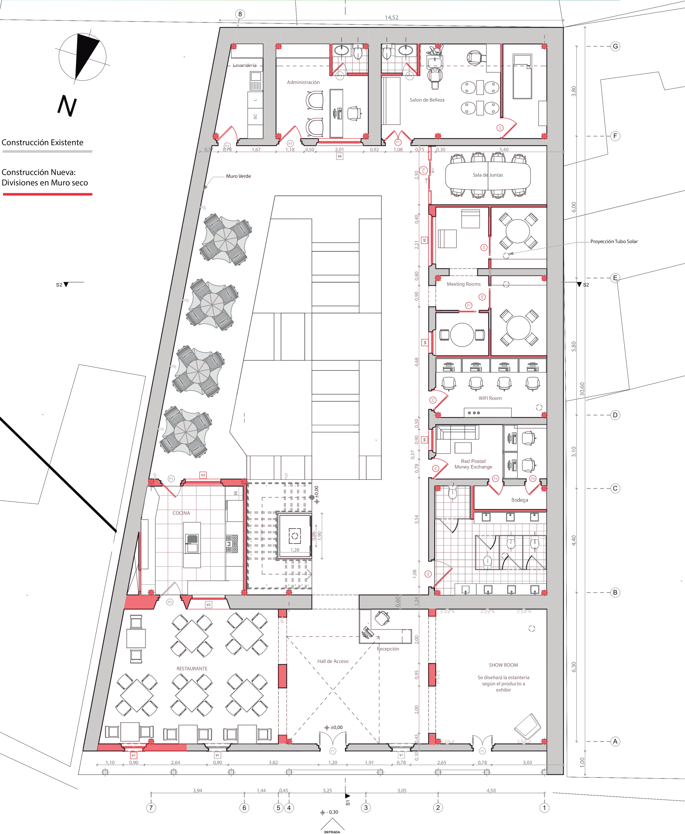
Calle 28 Planta Arquitectónica de Primer Piso
