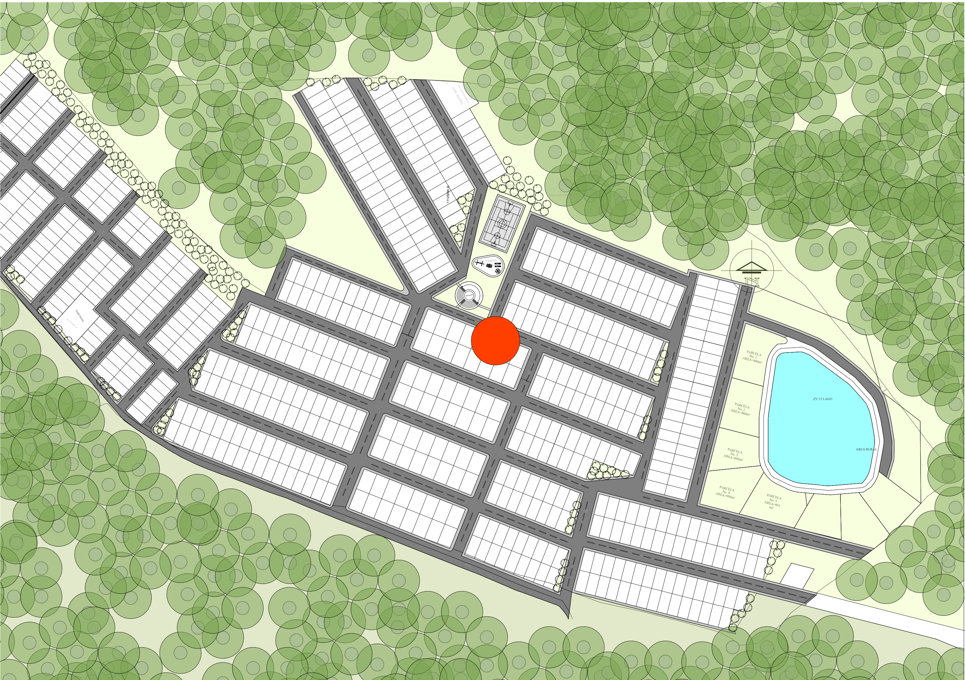
ESCALA MESO - ESC_1:1500 - URBANIZACION EL LIBANO
