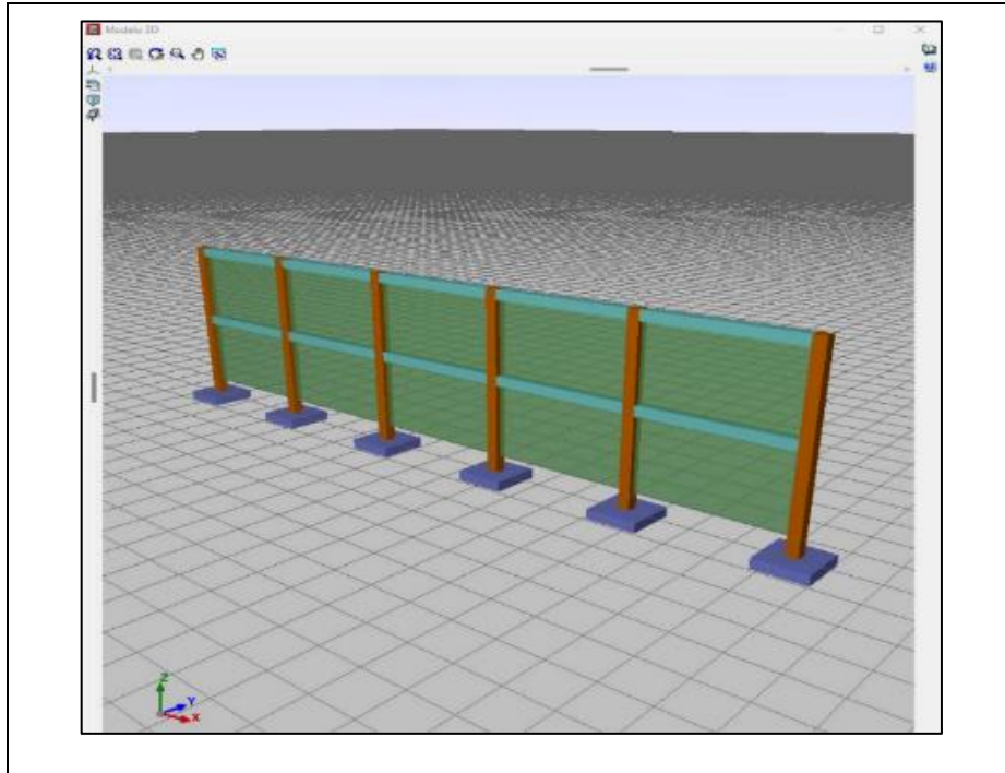
Modelación pórtico Software CYPECAD
