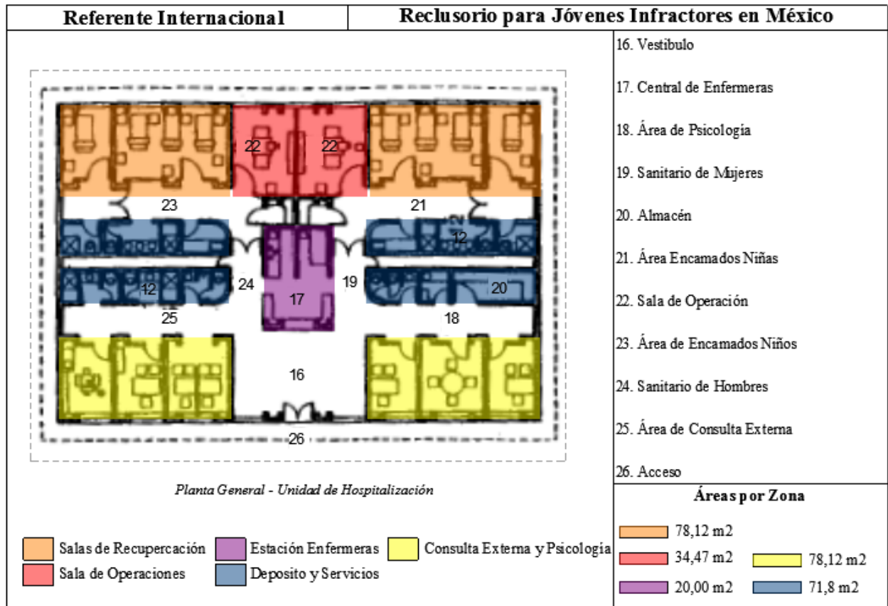
Figura 38. Planta Modulo de Hospitalización del Reclusorio, Adaptado de: Enciclopedia de Arquitectura Plazola Vol. 9
