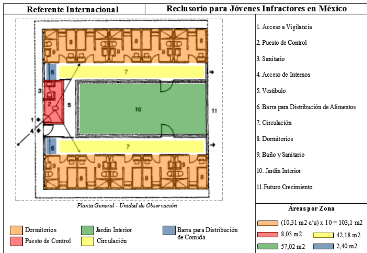
Figura 37. Planta Modulo de Hospitalización del Reclusorio, Adaptado de: Enciclopedia de Arquitectura Plazola Vol. 9
