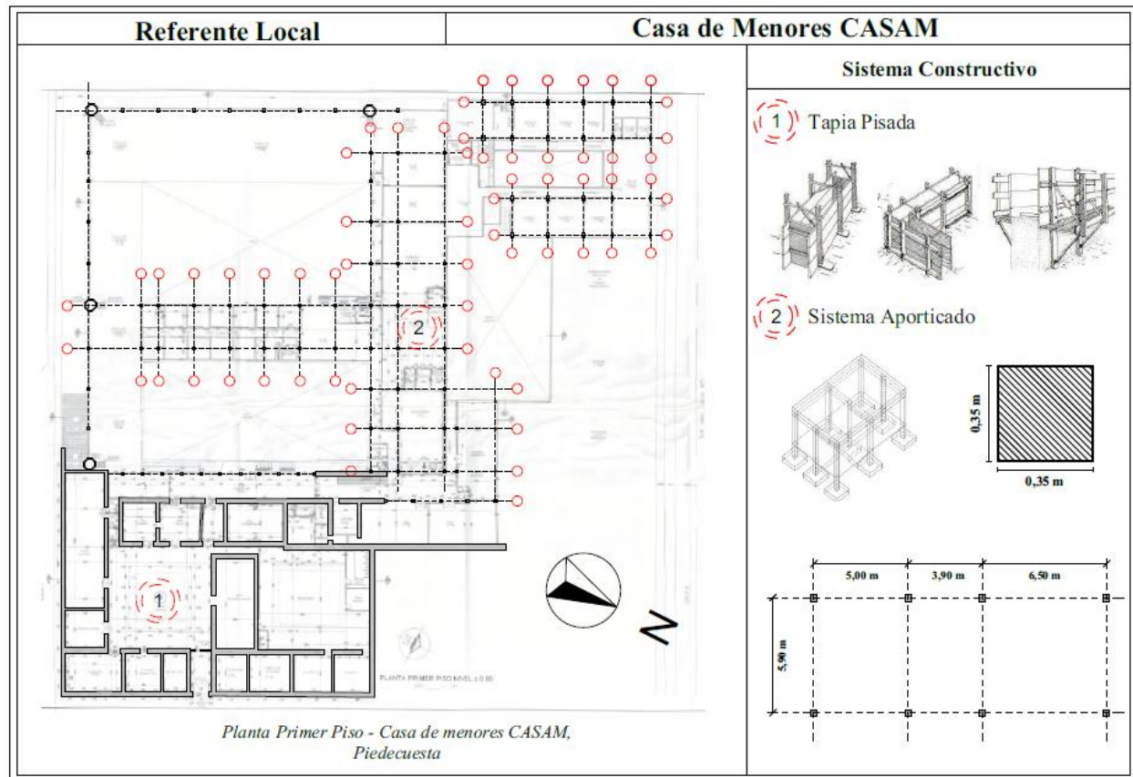
Figura 45. Sistemas constructivos empleados en la edificación, tapia pisada en la edificación inicial y sistema aporticado para las diferentes expansiones realizadas con el paso de los años
