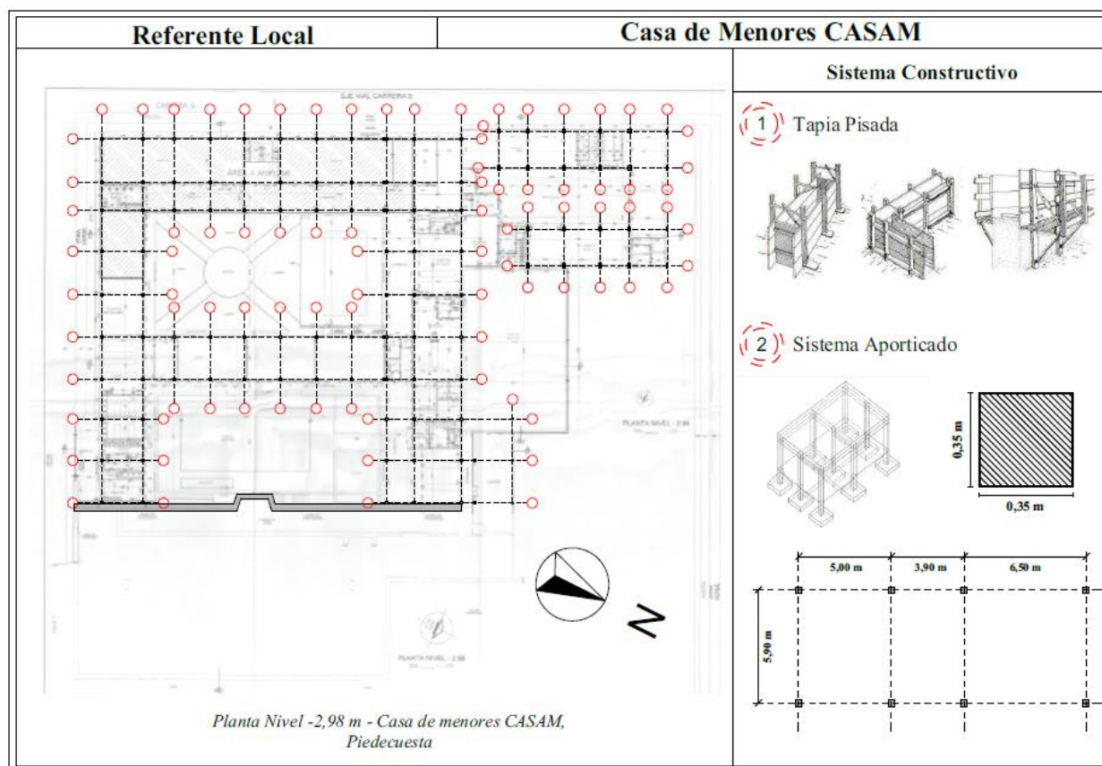
Figura 46. Sistemas constructivos empleados en la edificación, tapia pisada en la edificación inicial y sistema aporticado para las diferentes expansiones realizadas con el paso de los años
