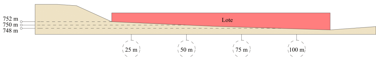
Figura 11. Corte del terreno, Adaptado de: Propio del Autor
