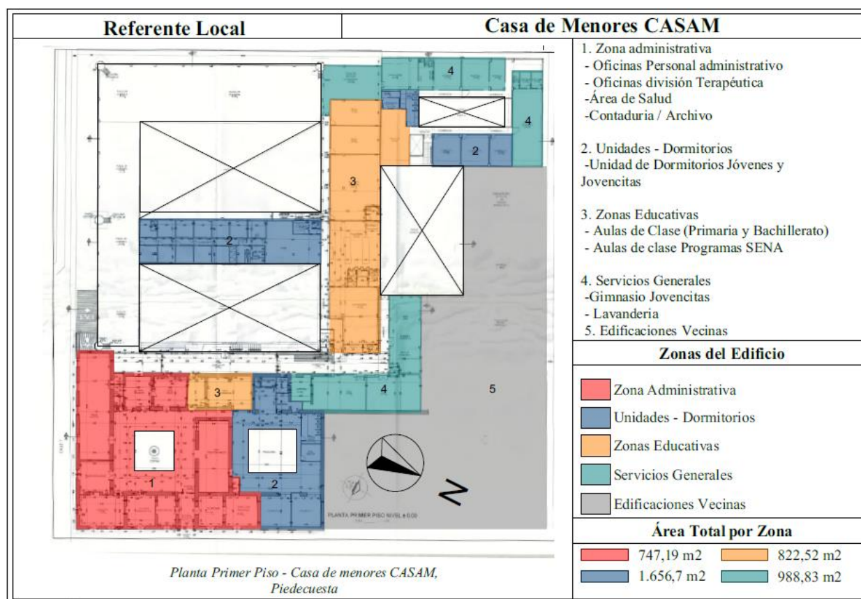
Figura 41. Casa de Menores CASAM, Panta de Primer piso, Adaptado de Dirección General del Centro de Atención Especializada en Piedecuesta
