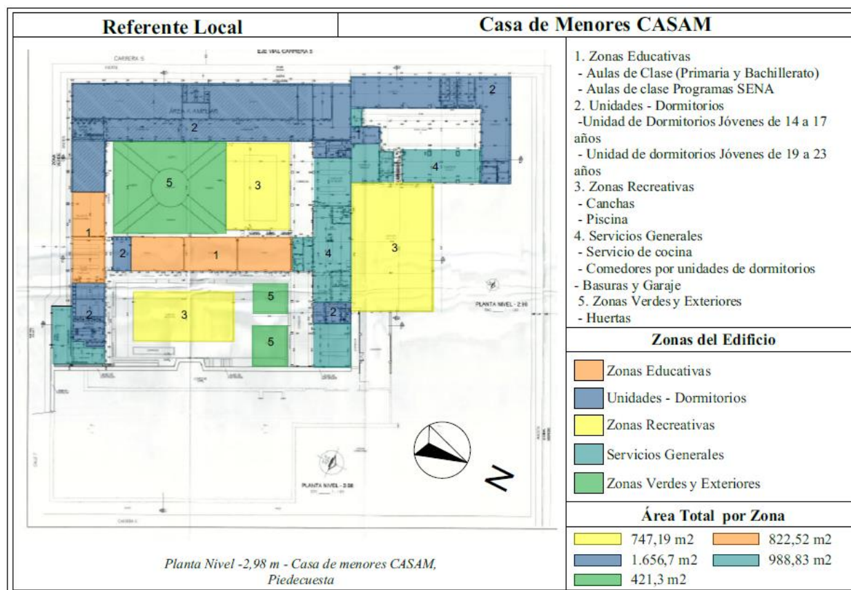
Figura 42. Casa de Menores CASAM, Planta nivel -2,98m, Adaptado de: Dirección General del Centro de Atención Especializada en Piedecuesta
