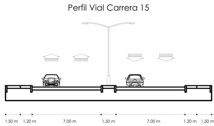
Figura 20. Perfil Vial Carrera 15, Adaptado de: Propio del autor
