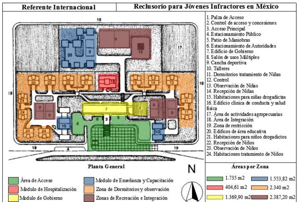
Figura 34. Planta General del Reclusorio, Adaptado de: Enciclopedia de Arquitectura Plazola Vol. 9
