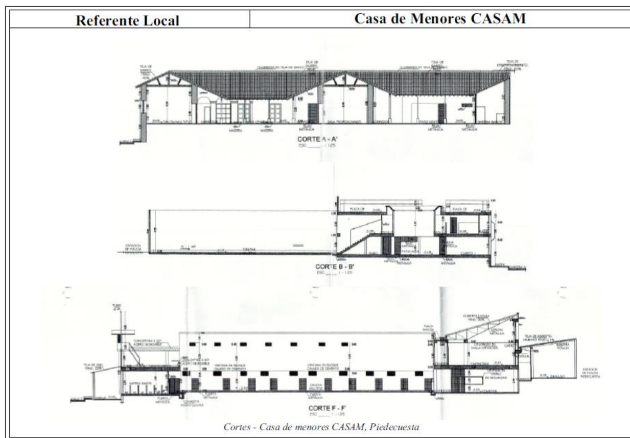
Figura 47. Cortes del Centro de Atención Especializada, Casa de Menores CASAM en Piedecuesta, Adaptado de: Dirección General del Centro de Atención Especializada
