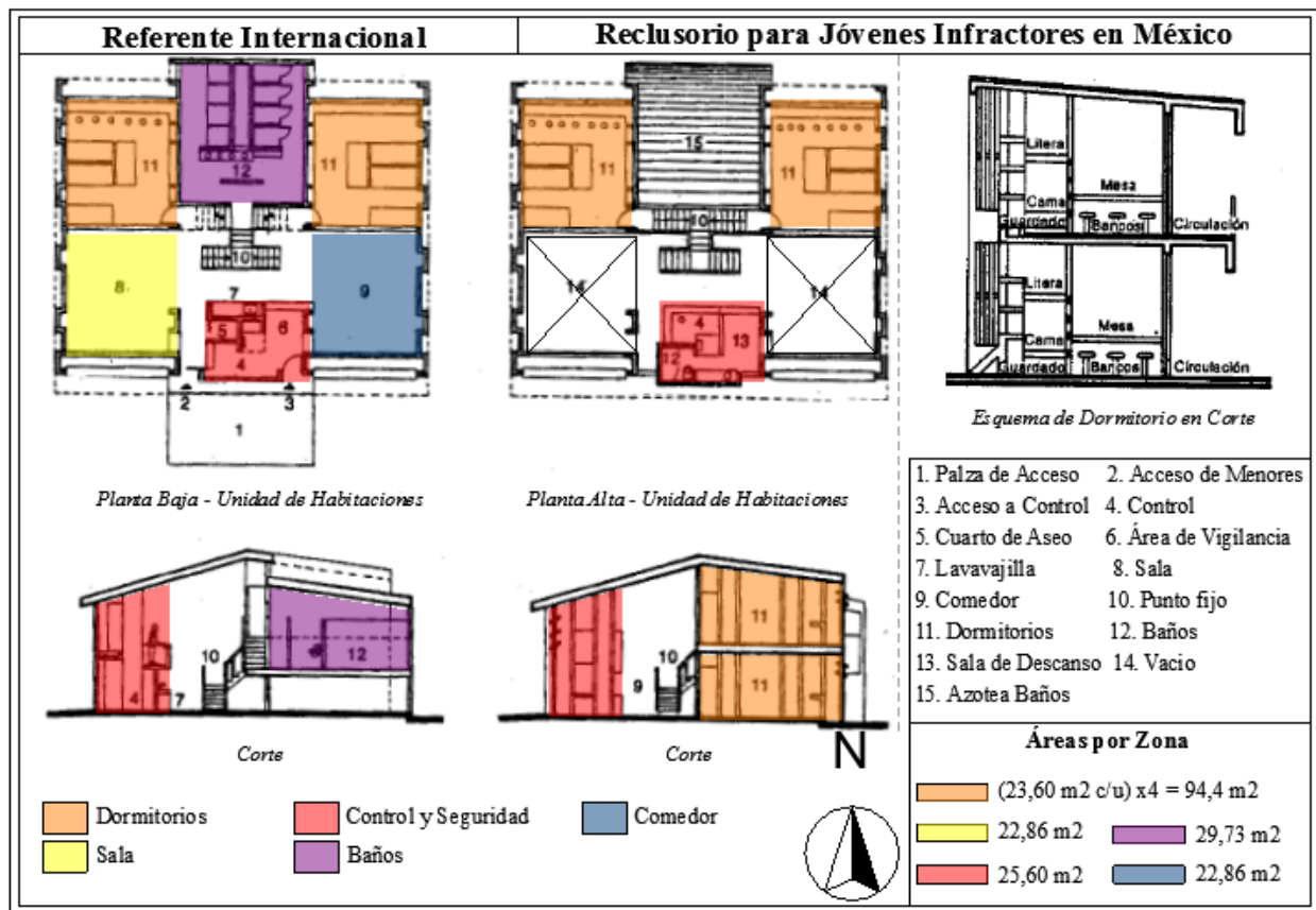
Figura 36. Plantas y Cortes de la Unidad de Habitaciones del Reclusorio, Adaptado de: Enciclopedia de Arquitectura Plazola Vol. 9
