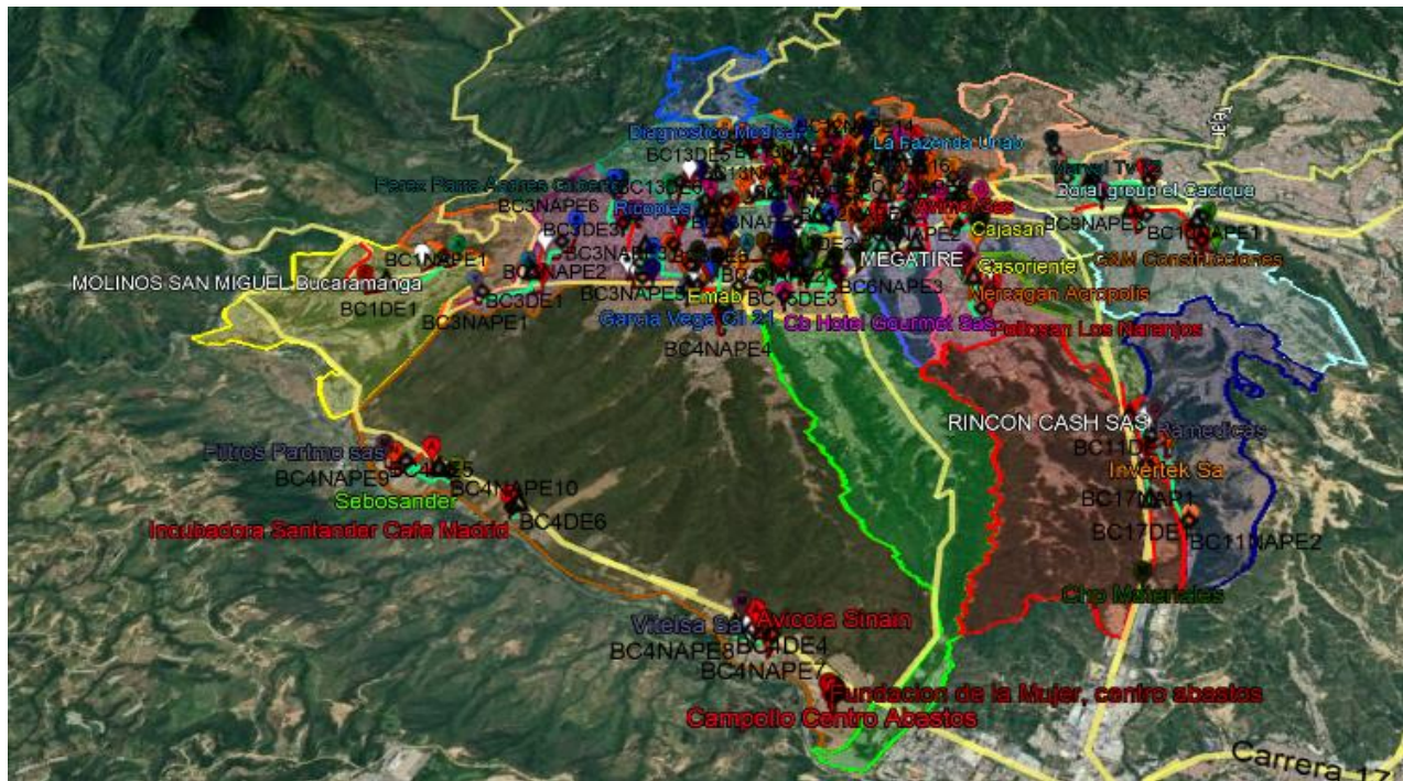
Figura 1. Diseño red FTTX -PON ciudad Bucaramanga.
