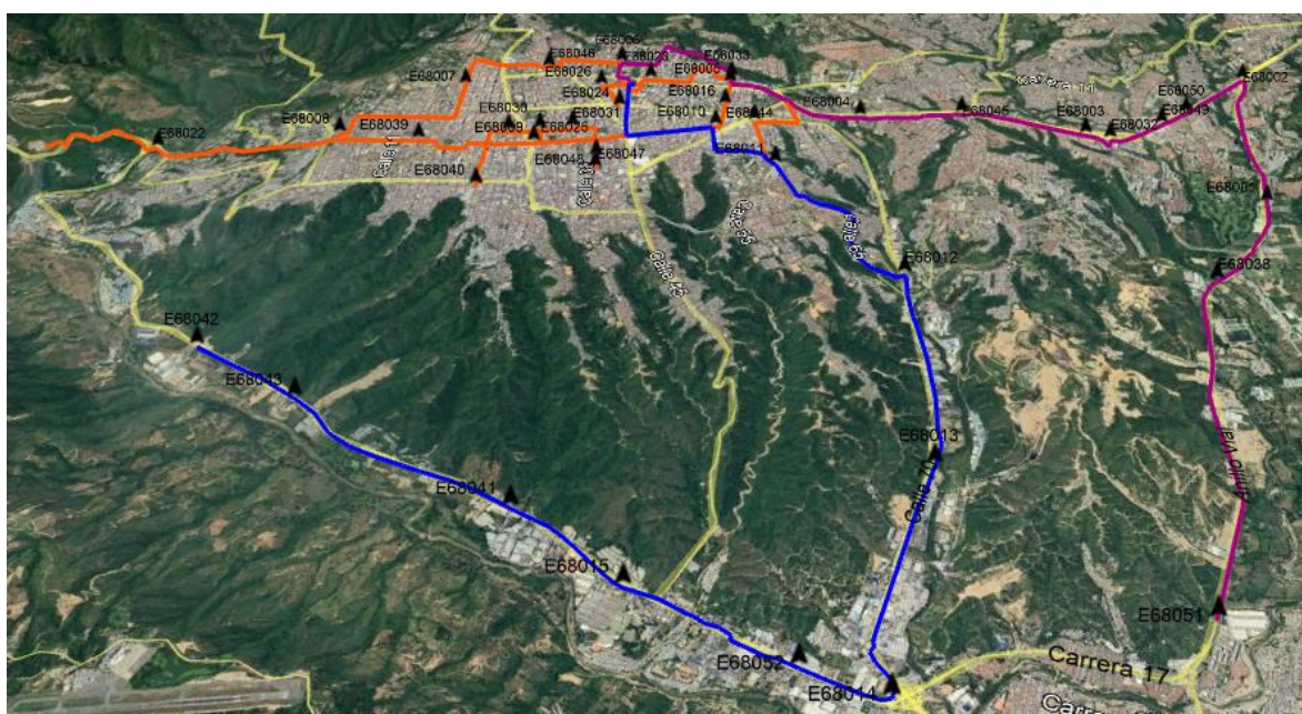
Figura 4. Red de Alimentación, Troncales de Alimentación y Cajas de Derivación
