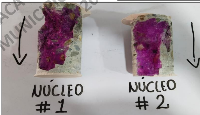
PRUEBA DE CARBONATACIÓN
