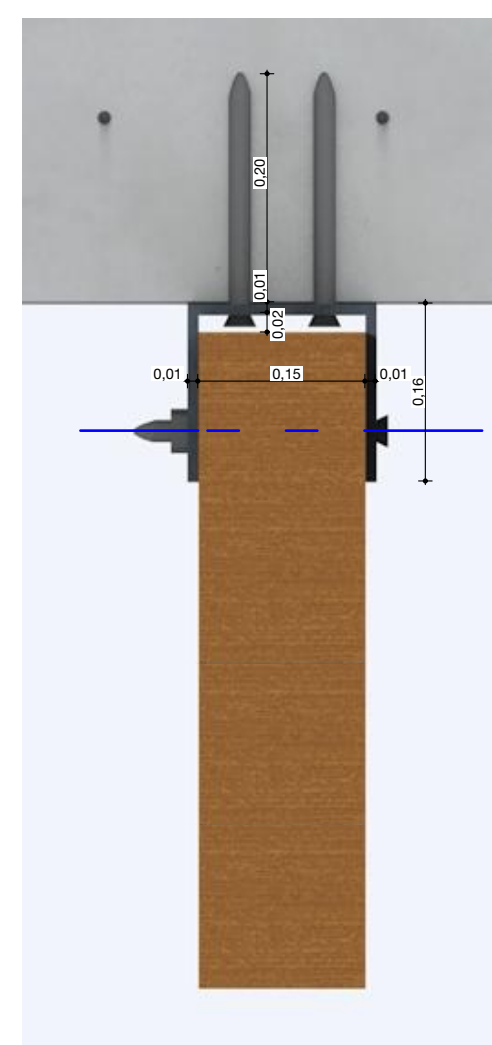
DETALLE ANCLAJE PARTESOLES
