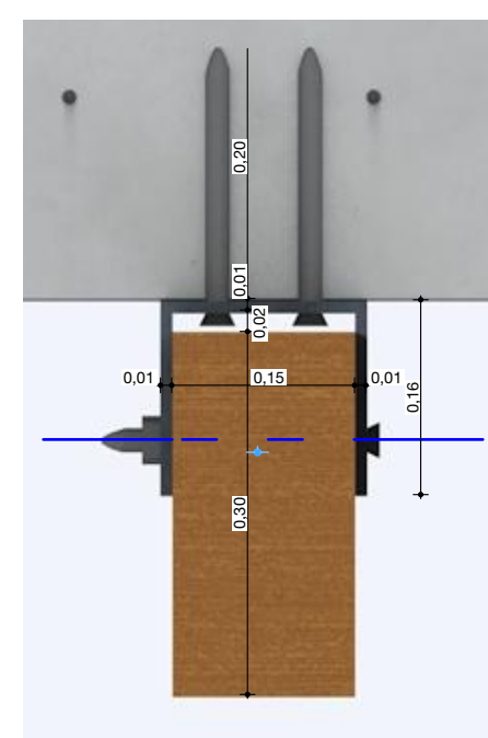
DETALLE ANCLAJE PARTESOLES
