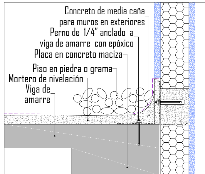
Imagen 99 - Detalle "C" - Conexión muro y media caña
