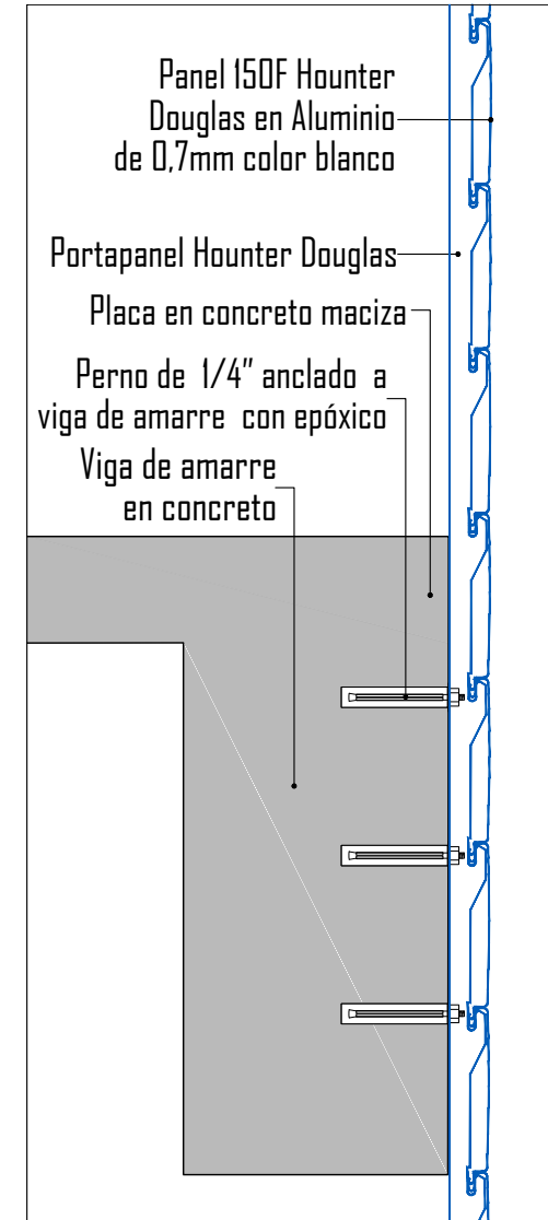
Imagen 98 - Detalle "B" - Fachada Hounter Douglas
