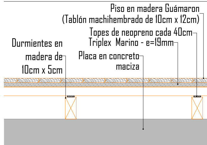
Imagen 97 - Detalle "A" - Piso en madera
