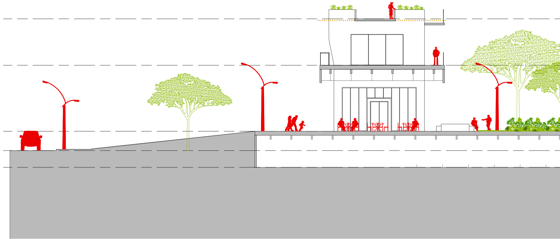
Corte B-B
