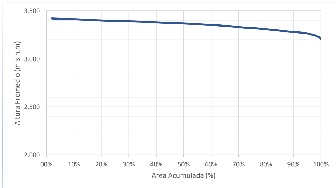
Figura 1-3 Curva Hipsométrica Fuente. Consorcio Aguas de los Andes, 2018
