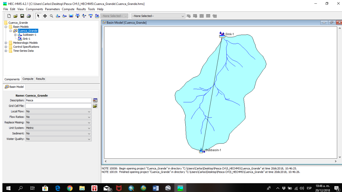
Figura 3-9 Cuenca Grande, HEC-HMS Fuente. Consorcio Aguas de los Andes, 2018
