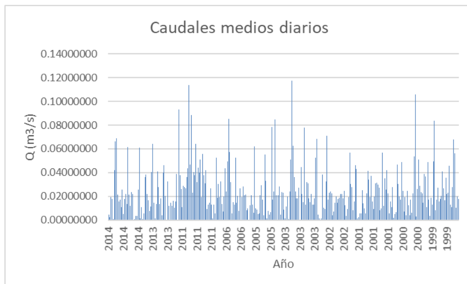
Figura 3-13 Caudales medios estimados, para la cuenca Grande Fuente. Consorcio Aguas de los Andes, 2018
