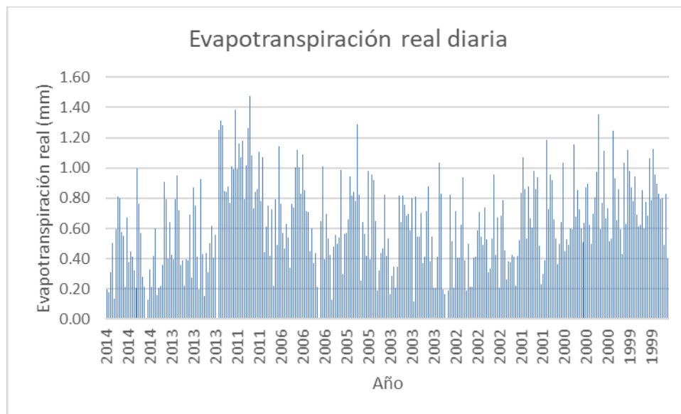
Figura 3-12 Evapotranspiración Real estimada para la cuenca Grande Fuente: Consorcio Aguas de los Andes, 2018
