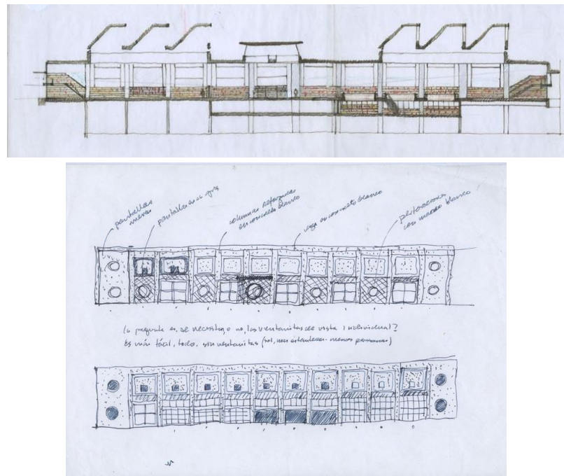
Figura 8. Bocetos de diseño. - archivo de la Biblioteca
