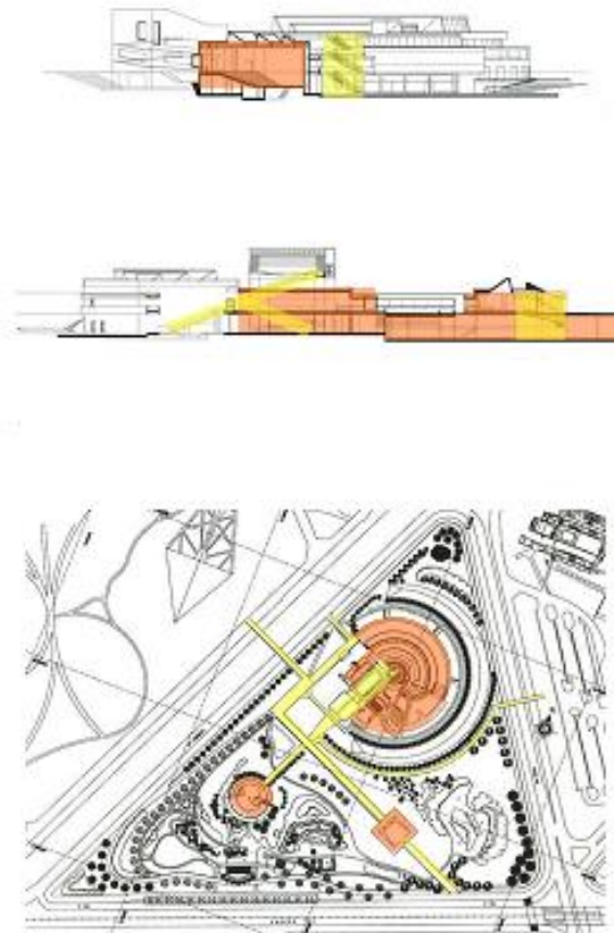
Figura 3. Cortes de la Biblioteca Virgilio Barco - archivo de la Biblioteca
