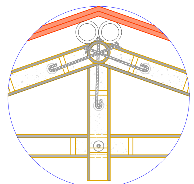
UNION ELEMENTOS DE CUBIERTA
