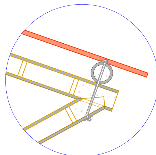
UNION ELEMENTOS DE CUBIERTA
