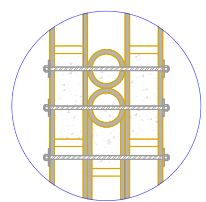
UNION TIPICA MONTANTE INTERMEDIO Y ARCO DE CARGA
