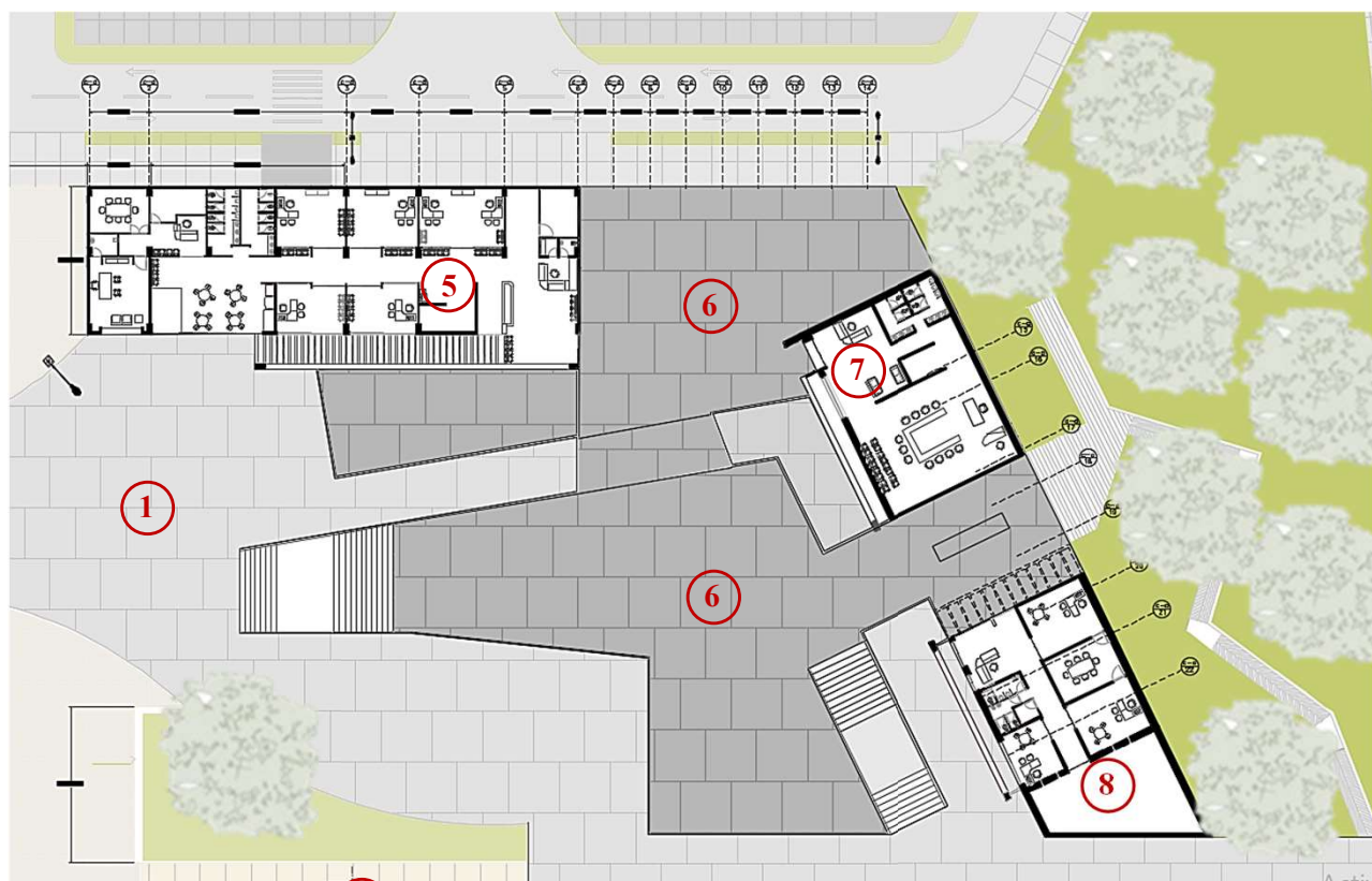
Imagen 60. Plantas arquitectónicas alcaldía, consejo municipal y juzgados
