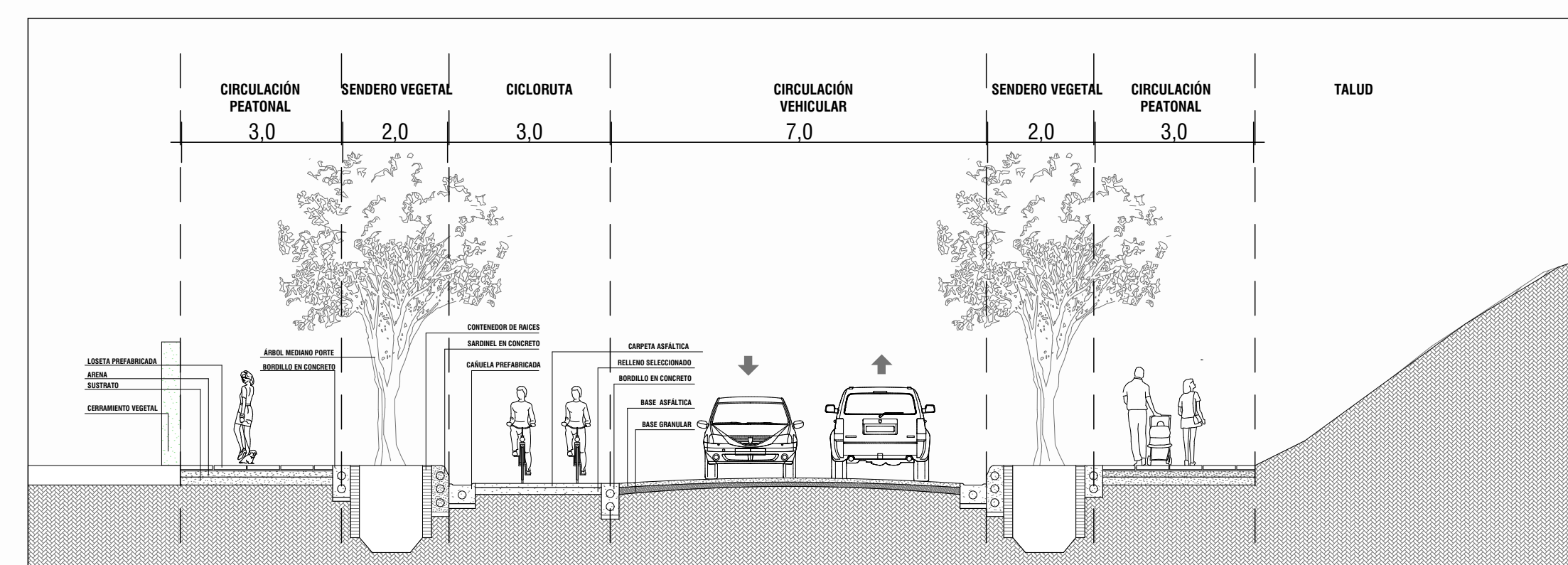
Perfil vial propuesta Esc_1:100
