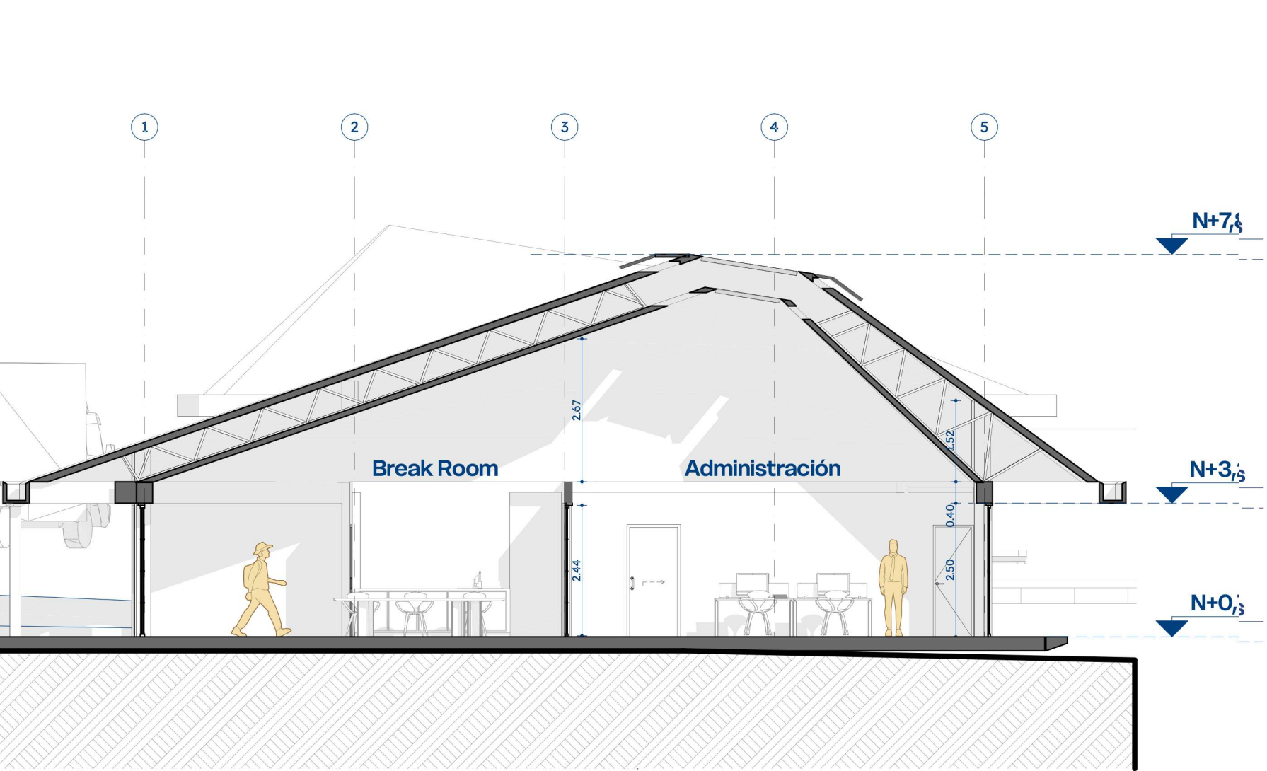
Sección S14-S14' Escala 1-100
