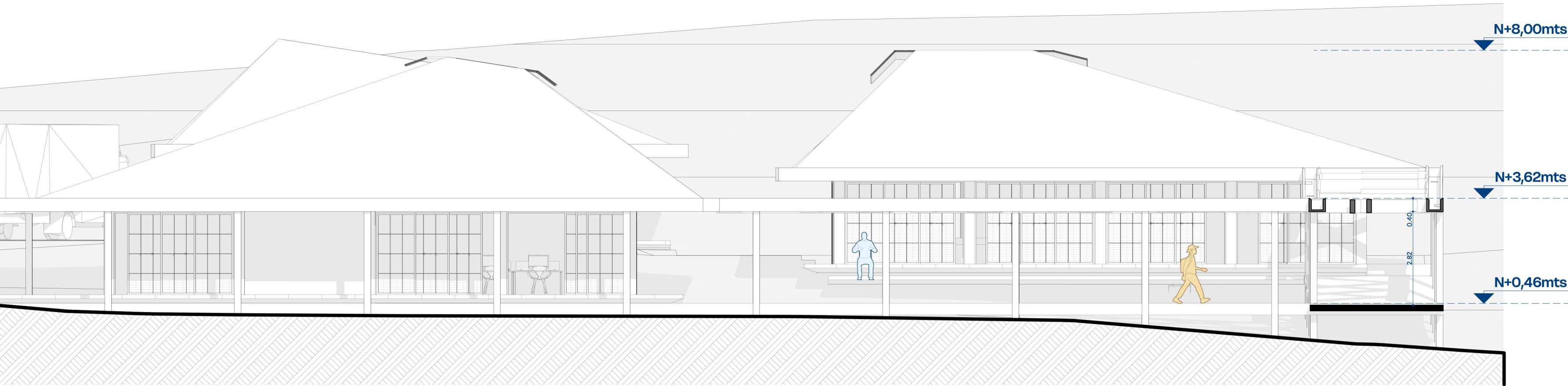
Sección S20-S20' Escala 1-100
