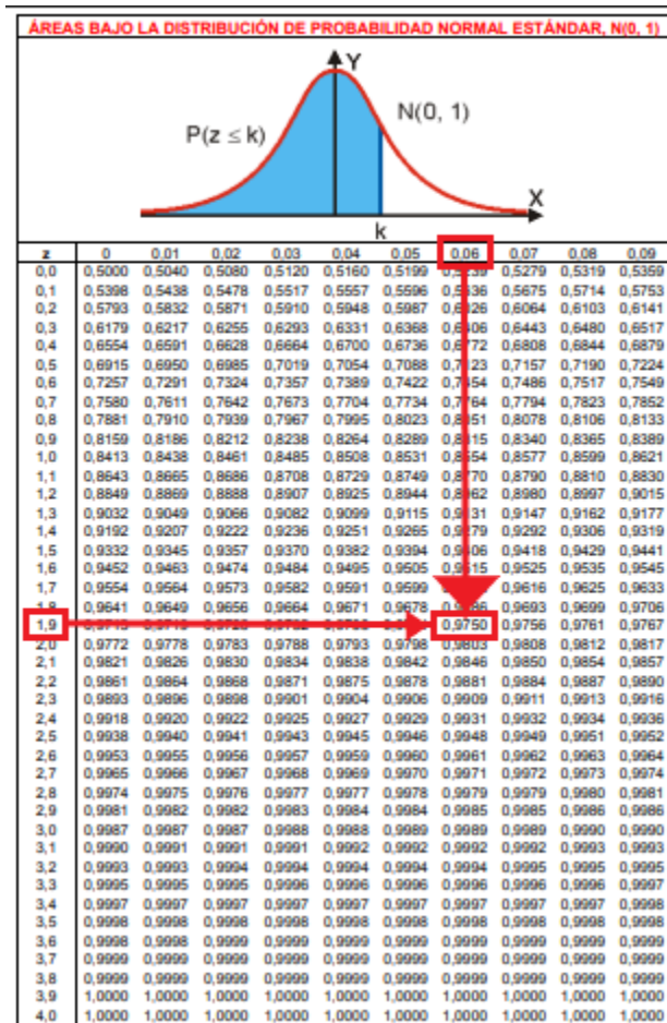
Figura 1. Distribución de probabilidad normal estándar.
