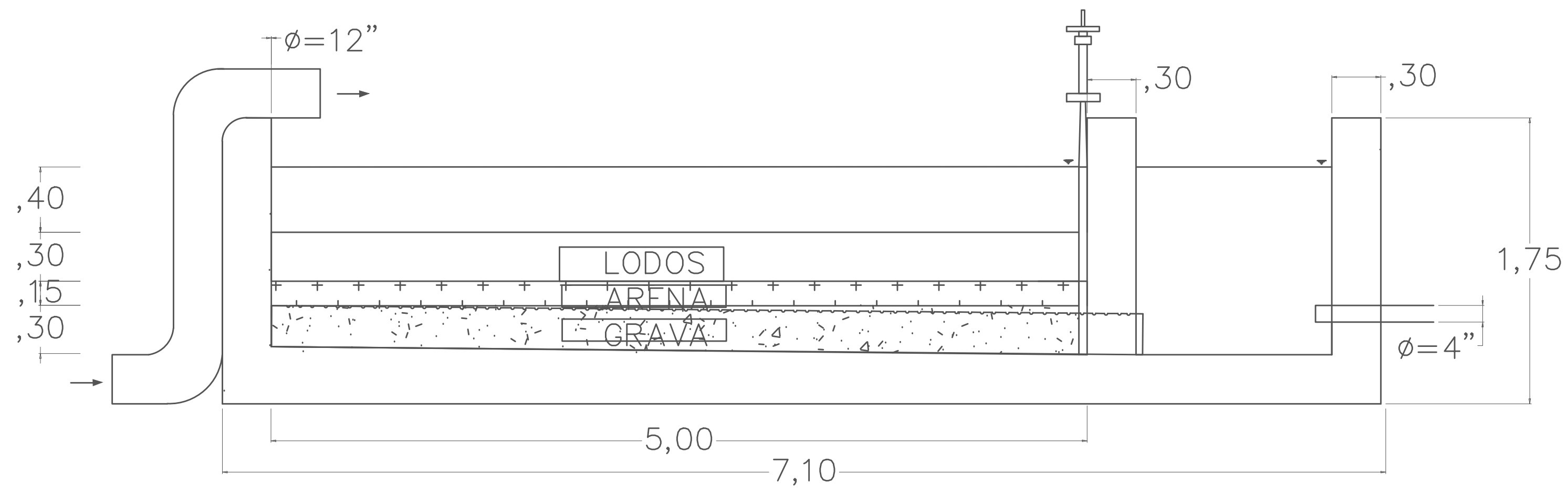
PERFIL LONGITUDINAL LECHO DE SECADO CORTE G—G
