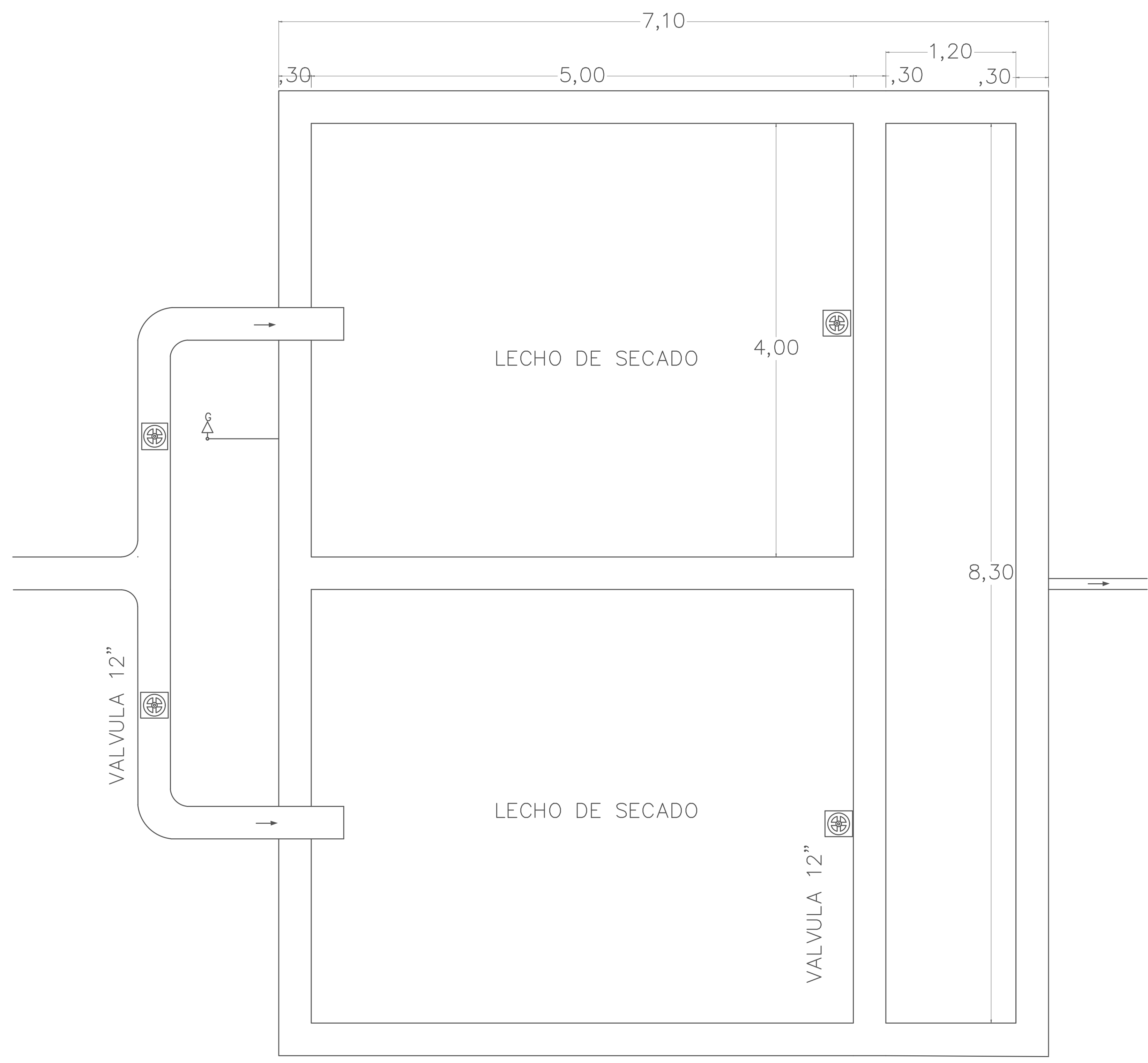
PLANTA LECHOS DE SECADO
