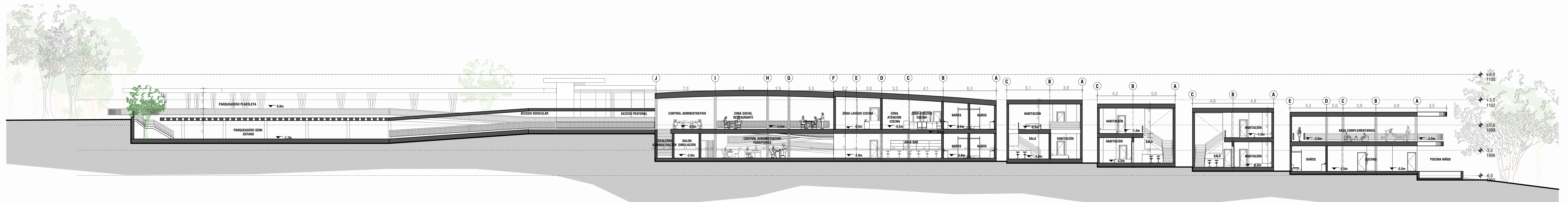
Sección Complejo G-G Esc 1:250
