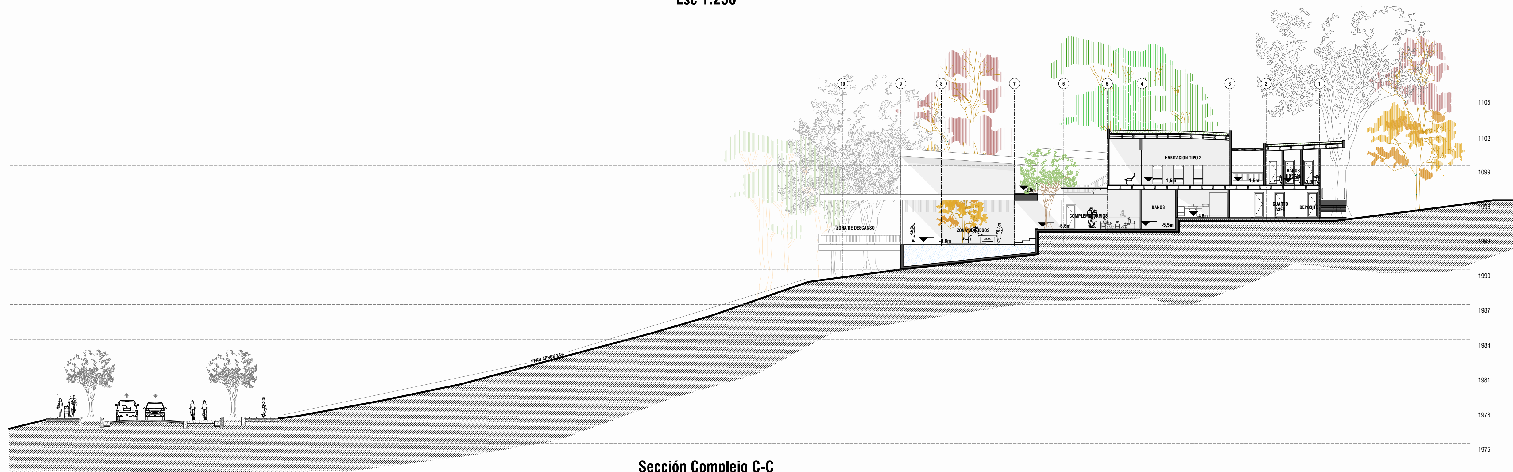
Sección Complejo C-C Esc 1:250
